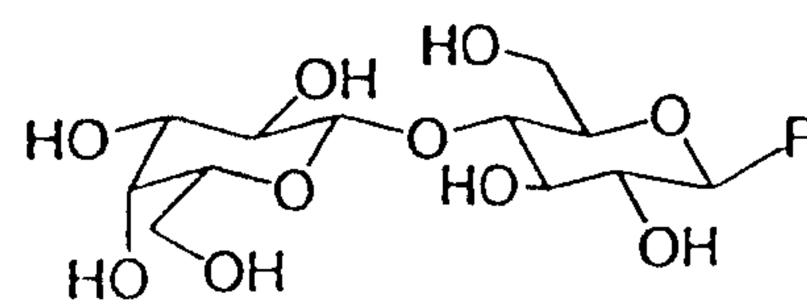
3. Lactose
