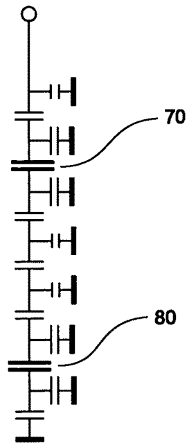
FIG. 28
