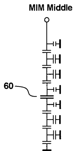
FIG. 25
