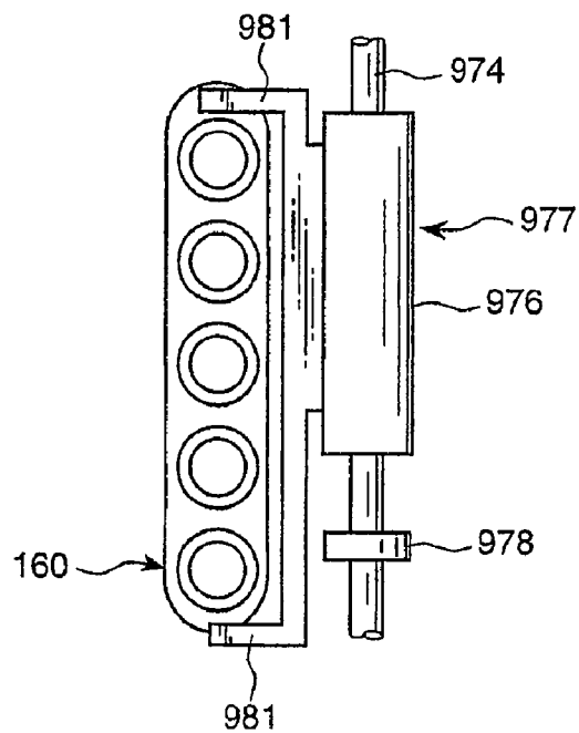
Fig. 42C
