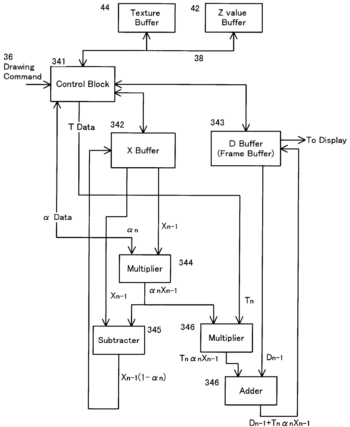
FIG. 5 Renderer
