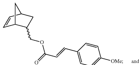
(bicyclo[2.2.1]hept-5-en-2-yl)methyl 3-(4-methoxyphenyl)acrylate (NBMeOCinnamate)
