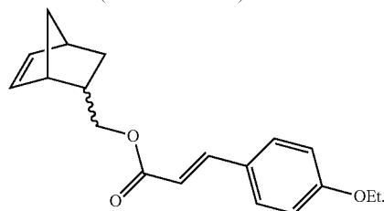
(bicyclo[2.2.1]hept-5-en-2-yl)methyl 3-(4-ethoxyphenyl)acrylate (NBEtOCinnamate)
