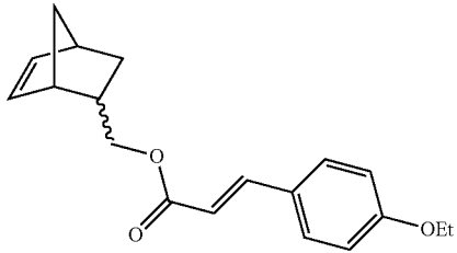
(bicyclo[2.2.1]hept-5-en-2-yl)methyl 3-(4-ethoxyphenyl)acrylate (NBEOCinnamate).
