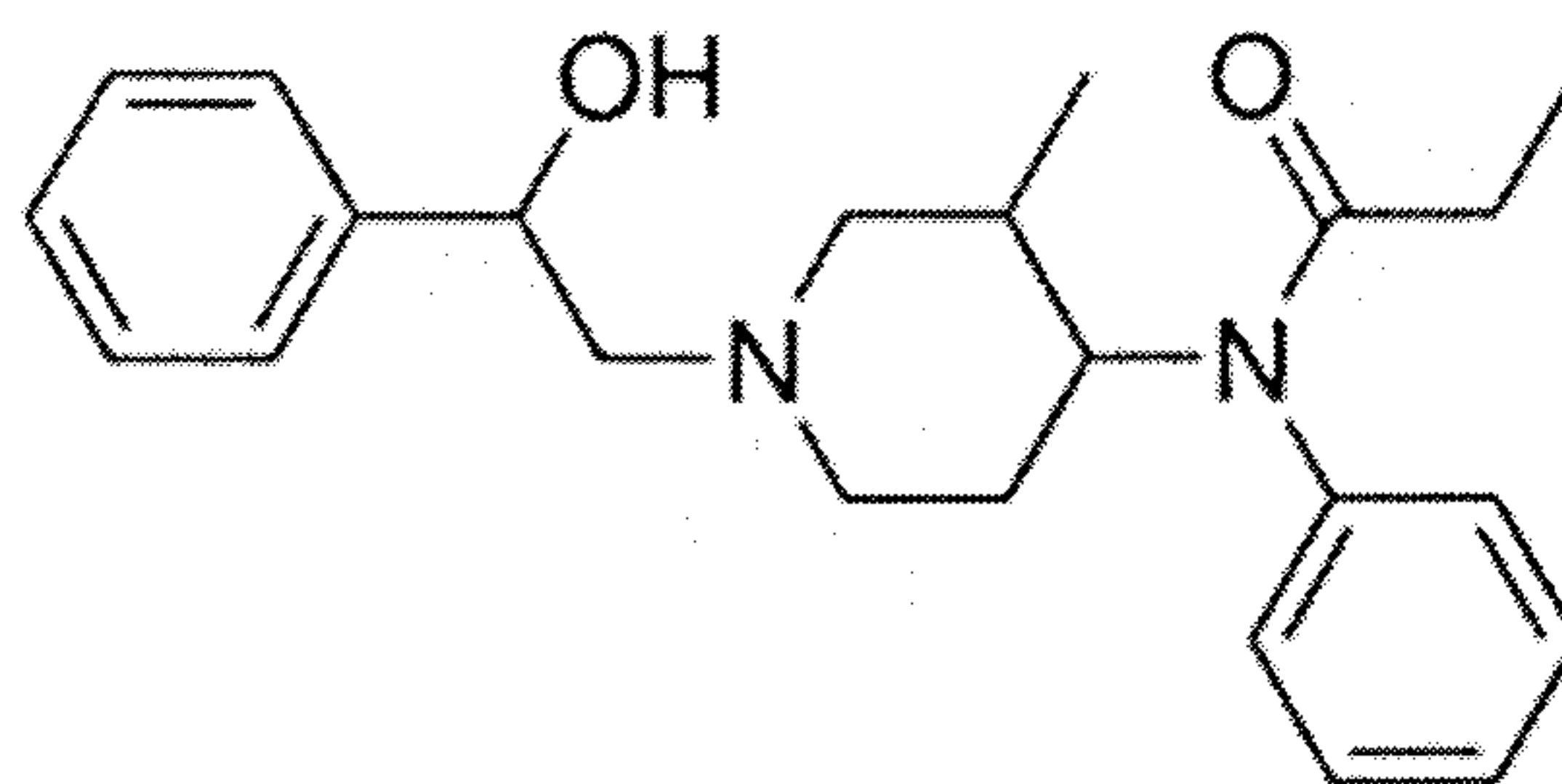
Ohmefentanyl
