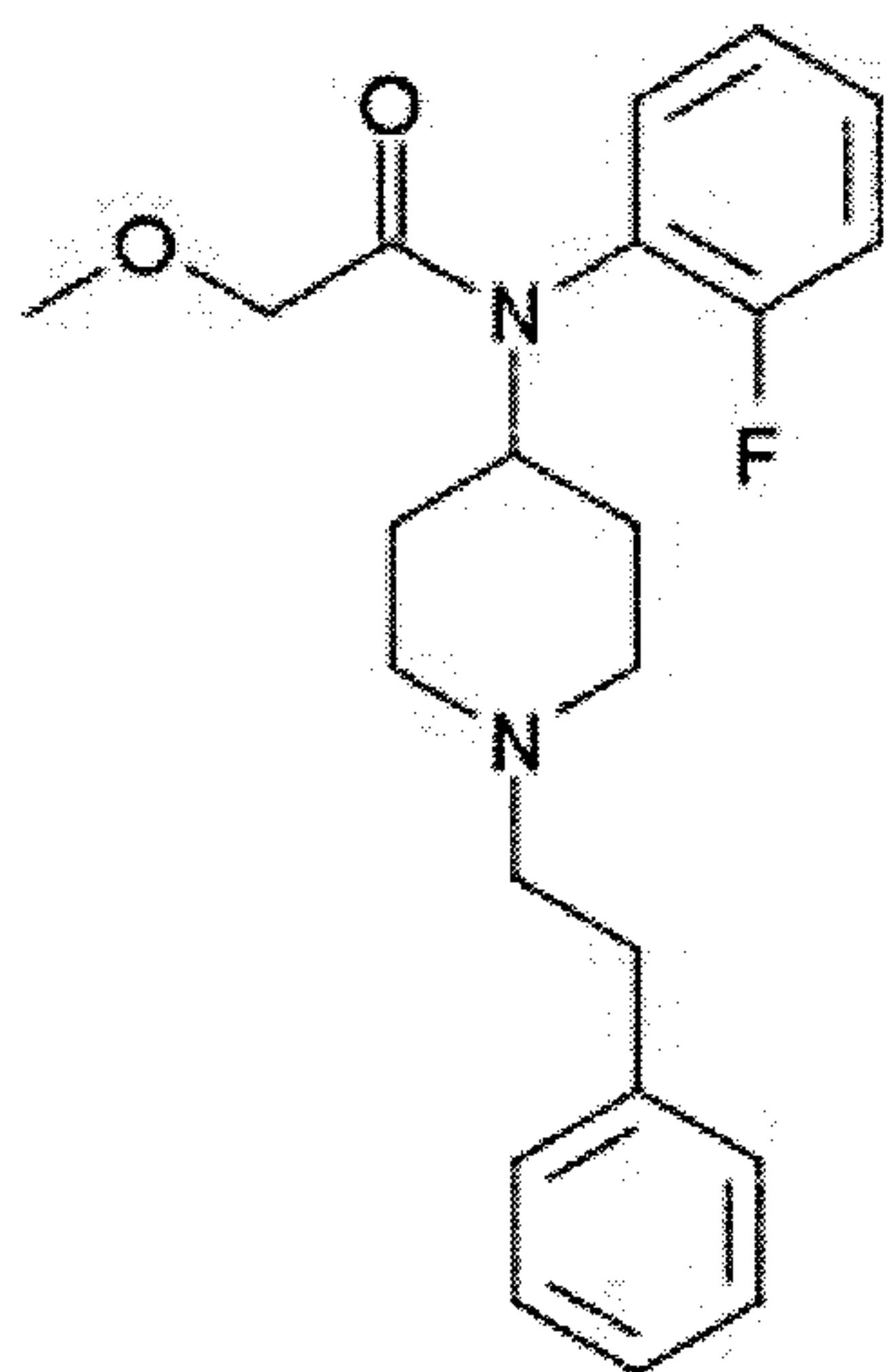
Methoxyacetylfentanyl
