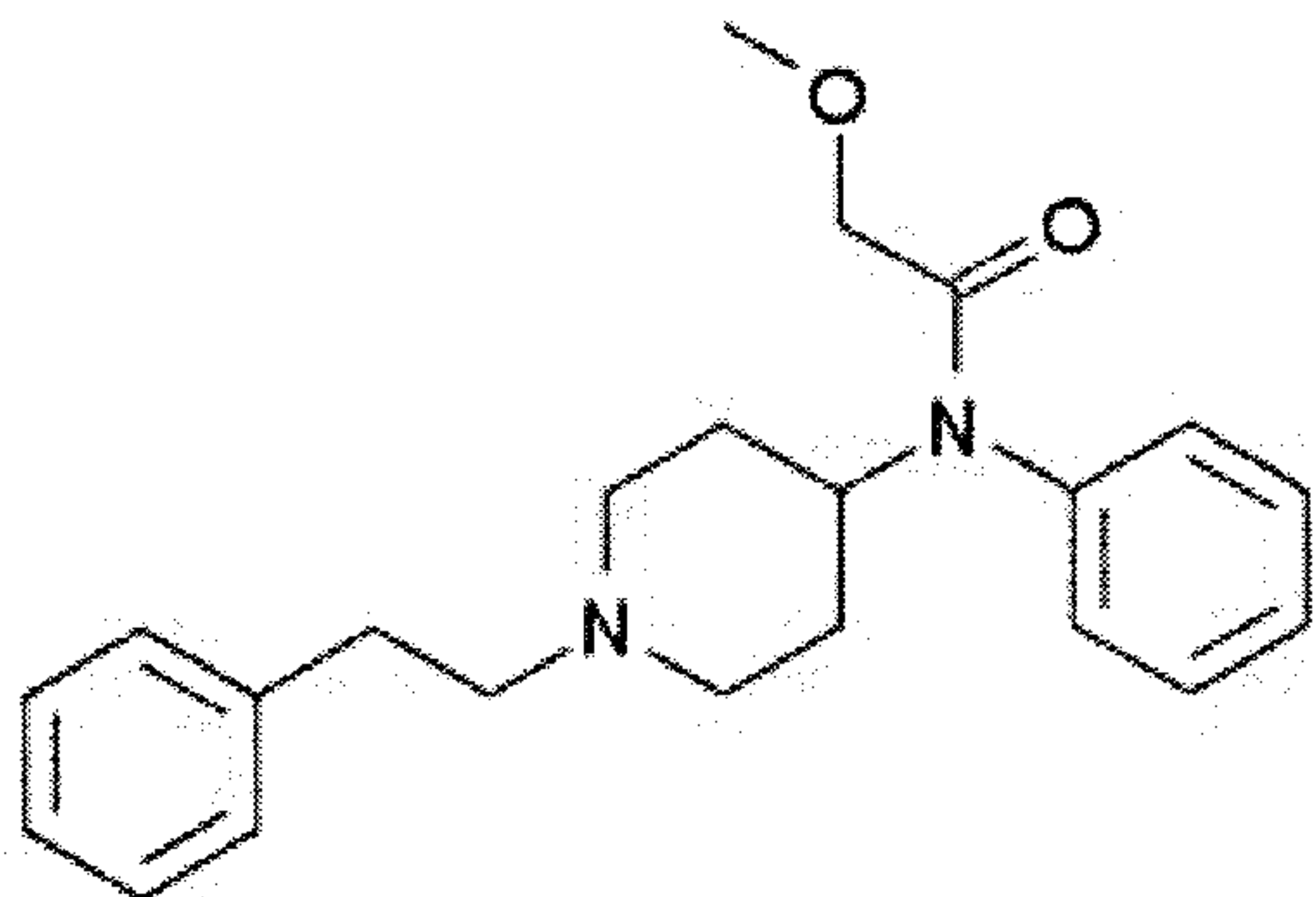
Methoxyacetylfentanyl
