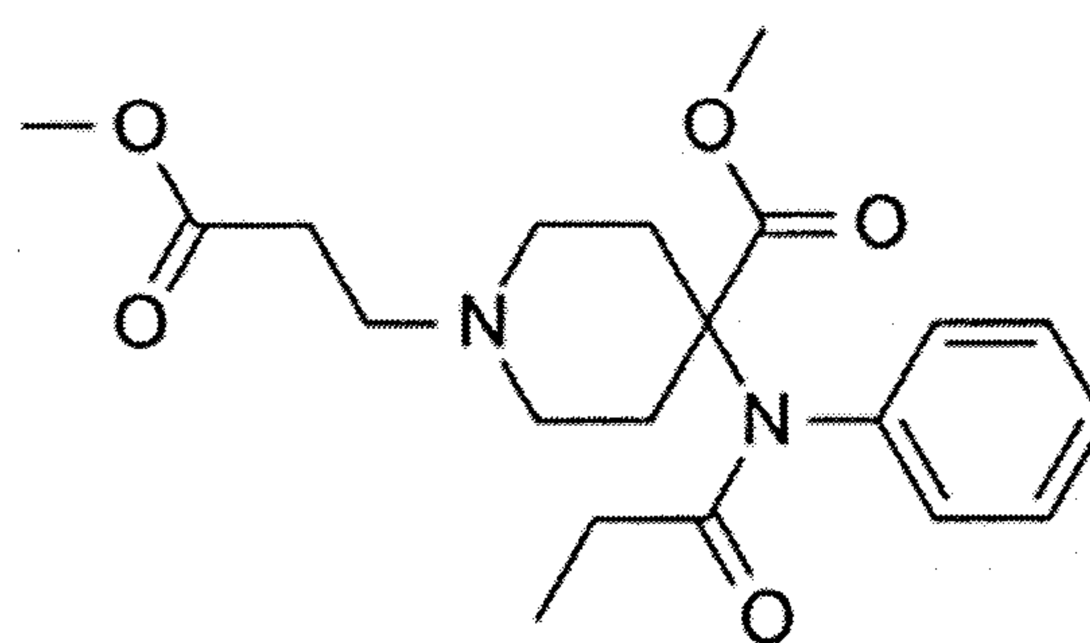
Remifentanyl
