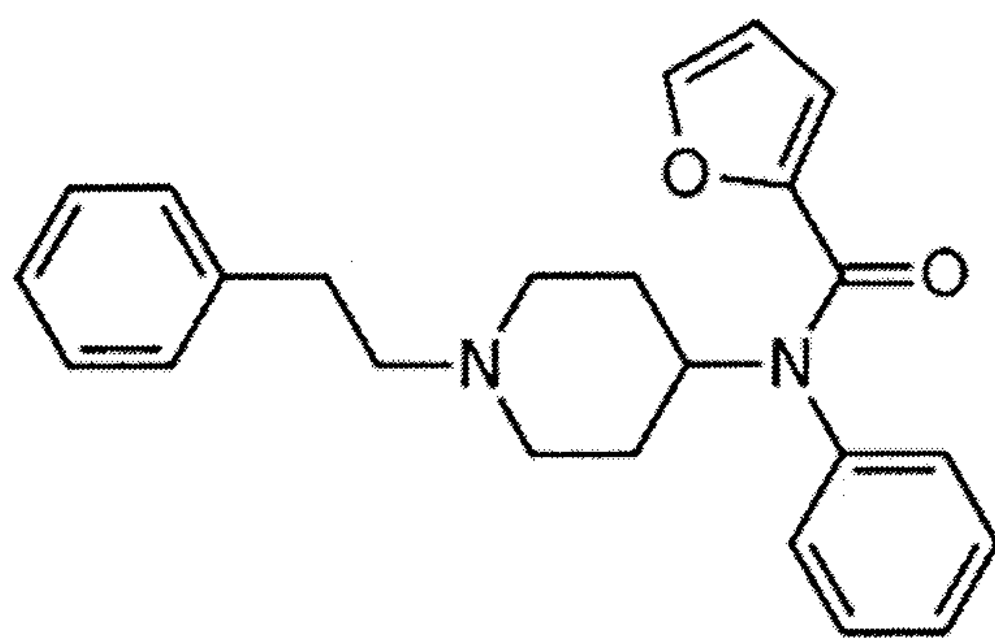
Furanylfentanyl
