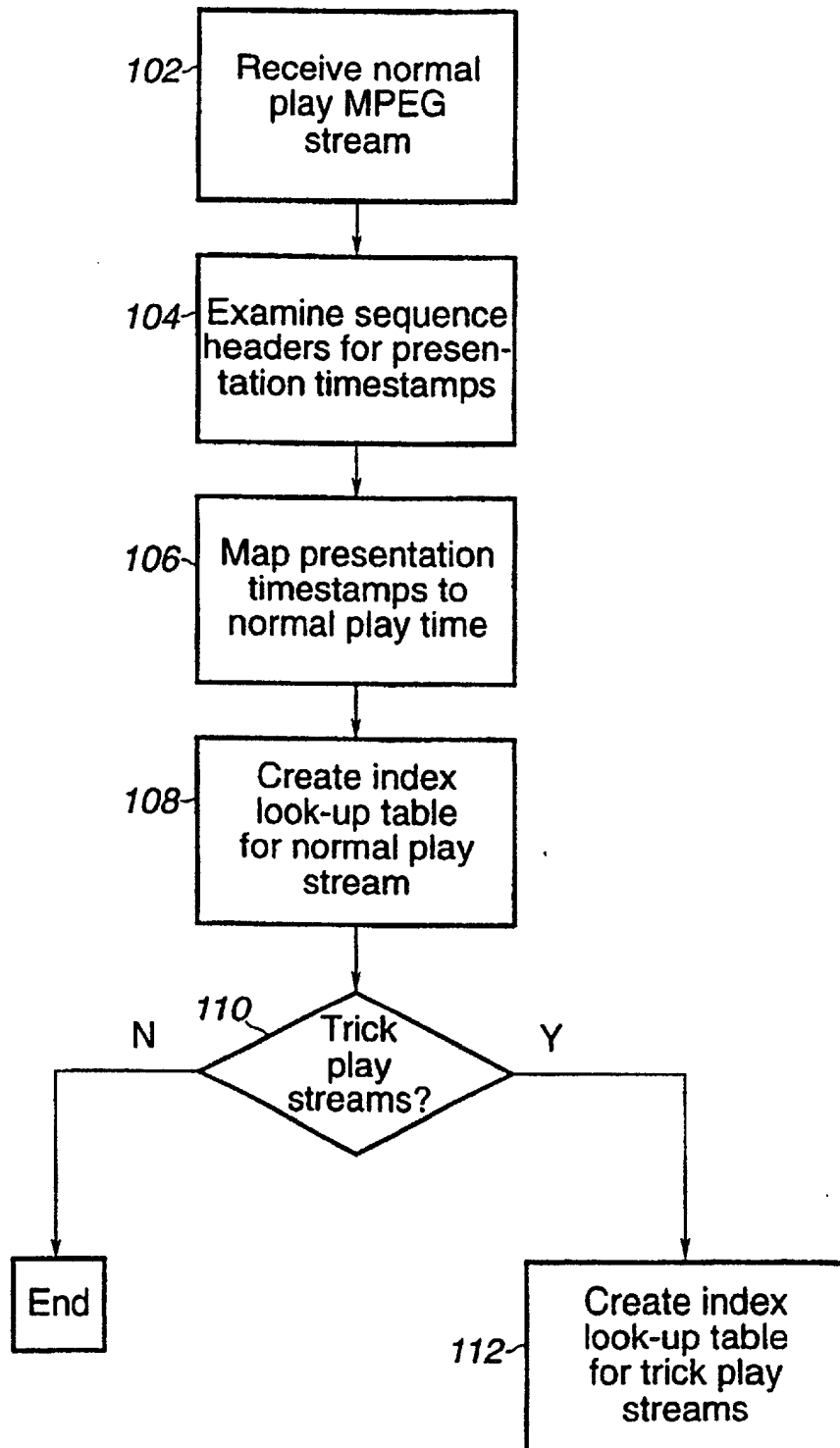
Fig. 5 Create Index table
