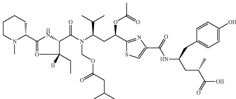
Tubulysin A
