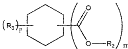
[Formule chimique 2]
