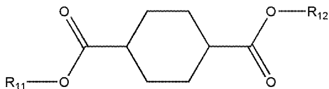
[Chemische Formel 1-1]
