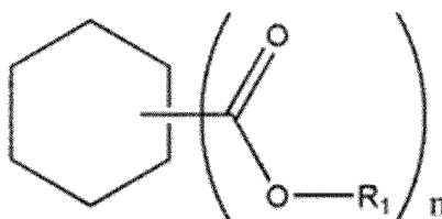
[Formule chimique 2]
