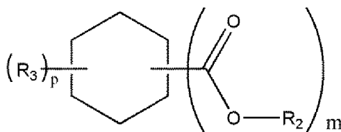
[Chemische Formel 2]
