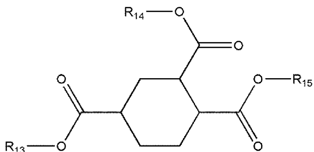
[Chemische Formel 1-3]
