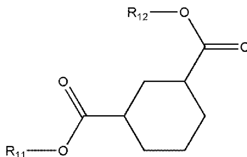
[Chemische Formel 1-3]
