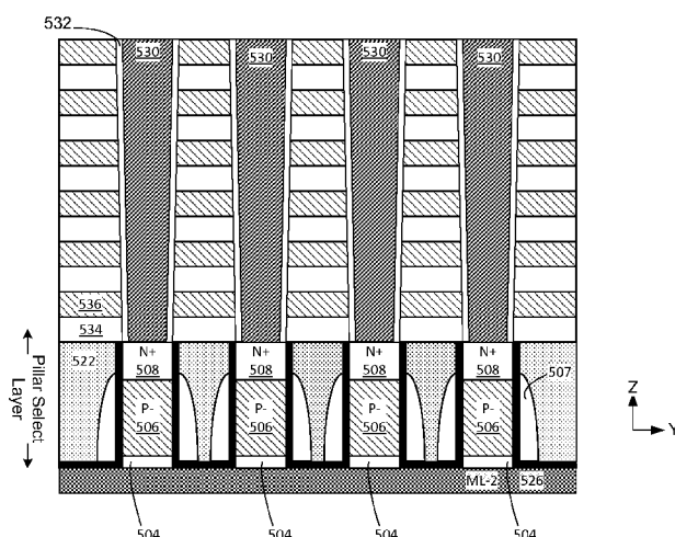
FIG. 14g
