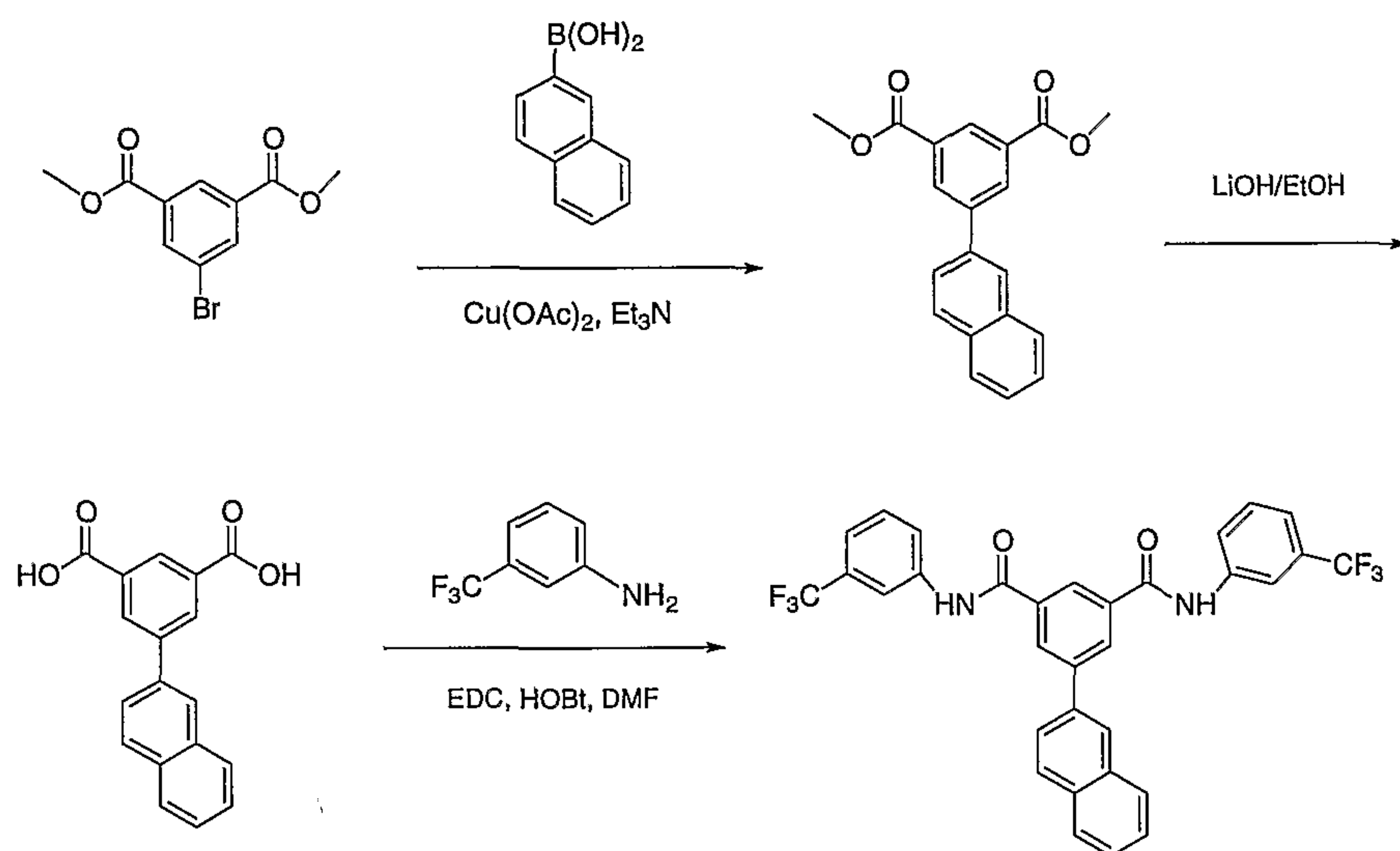
Scheme 1-E
