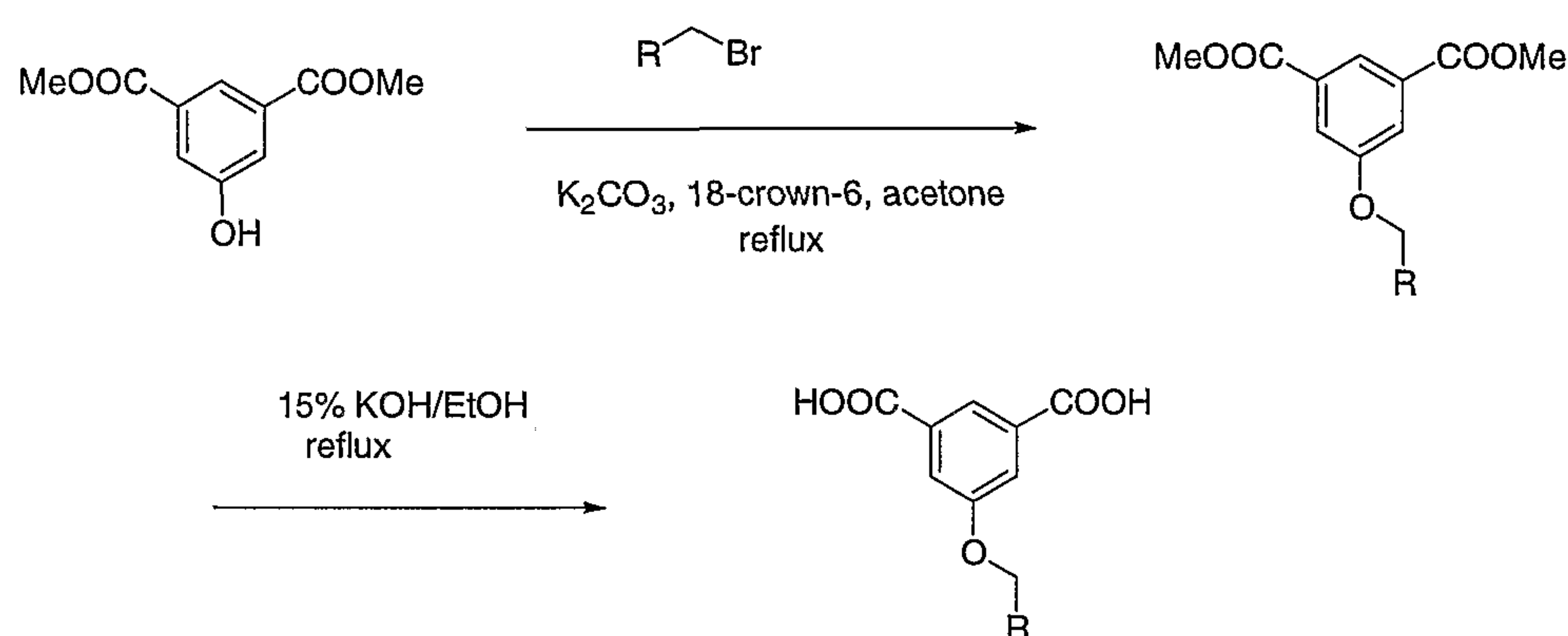
Scheme I-A
