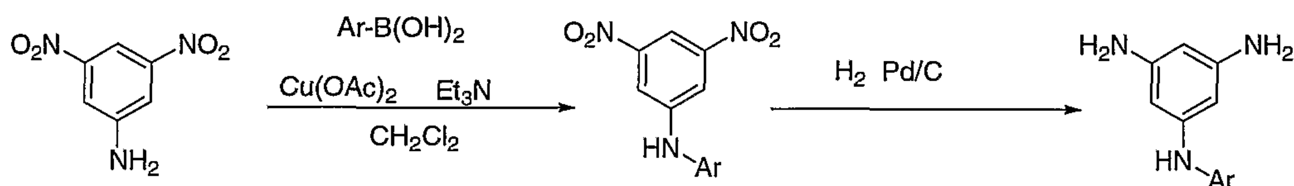
Scheme II-A
