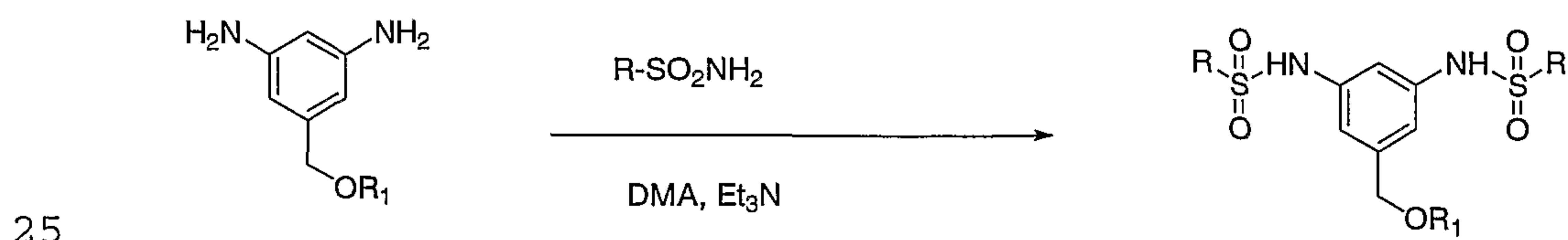
Scheme IV-A
