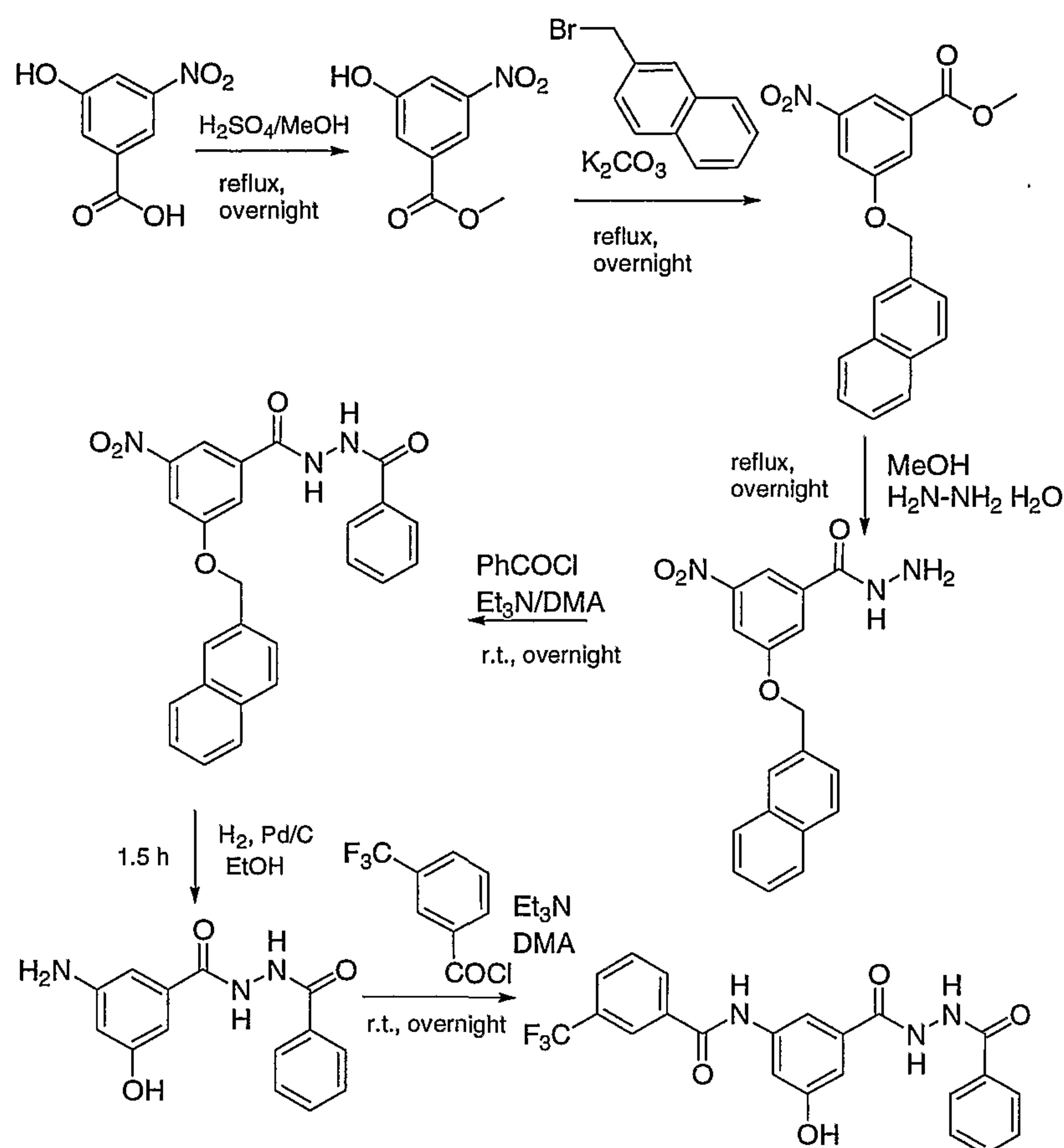
Scheme VI
