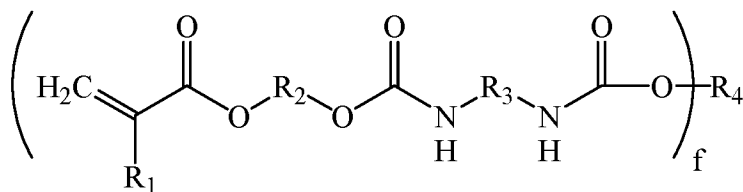
Formula A-I
