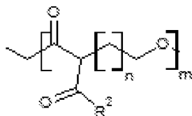
Formula D-VI
