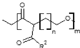
Formula D-VI
