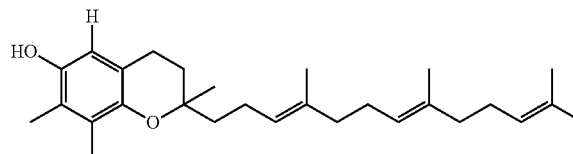
Gamma-tocotrienol
