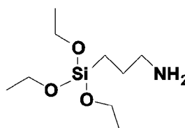
3-aminopropyl triethoxysilane
