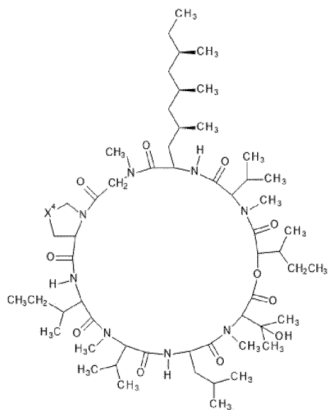
(I-B1)
