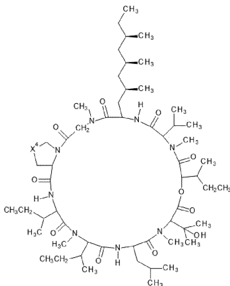
(I-B2)
