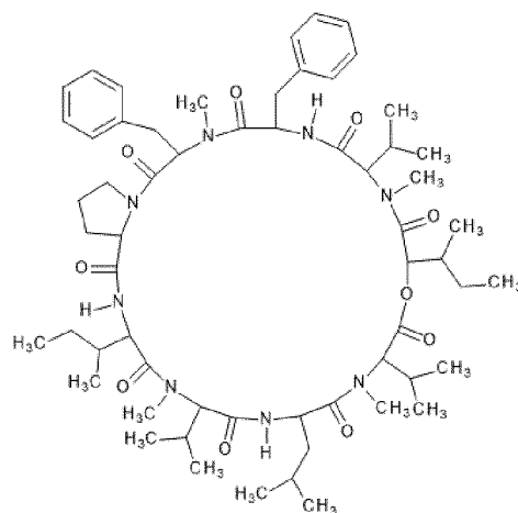
(I-A3)
