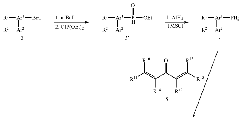
Scheme A'
