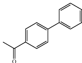
4-Acetylbiphenyl
