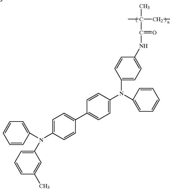
TPD-PMAA
