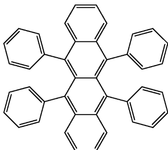
Rubrene
