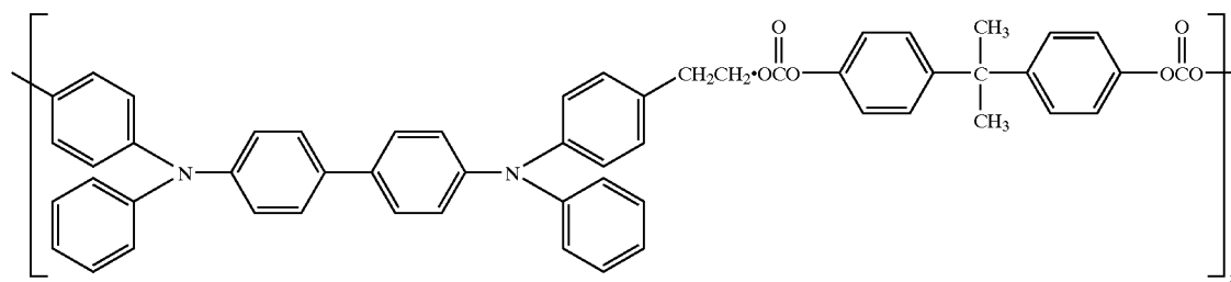
TPD-PCA
