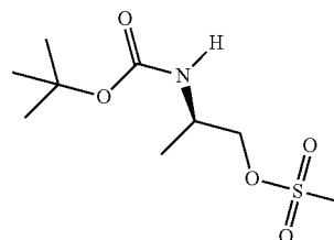
A. (R)-2-((tert-Butoxycarbonyl)amino)propyl methanesulfonate
