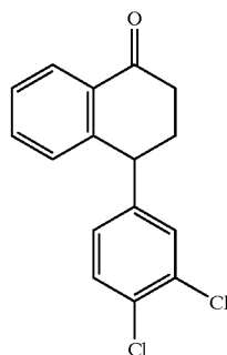
Sertralone
