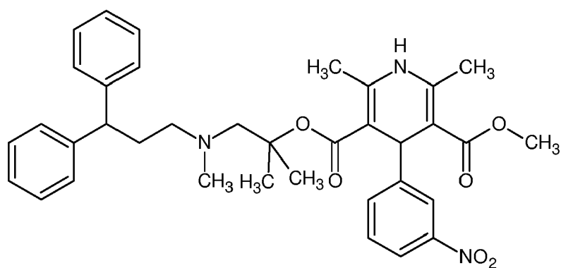
(I-c)
