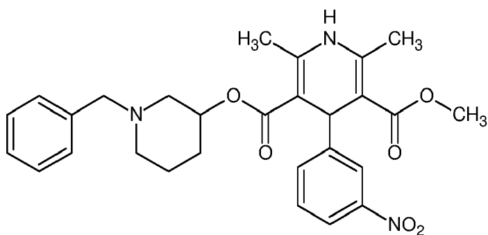
(I-f)
