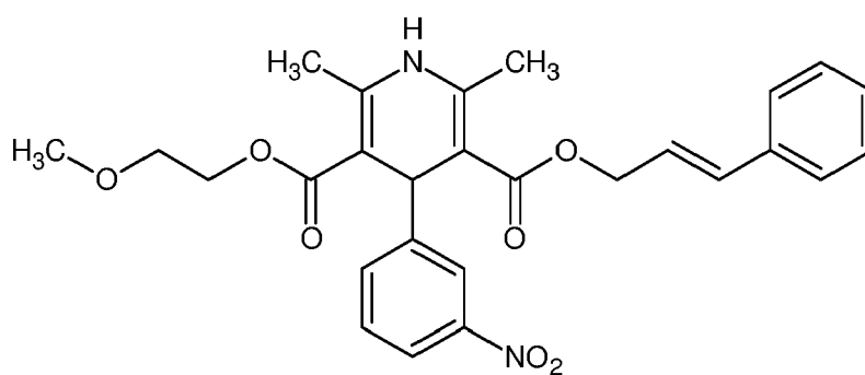
(I-b)
