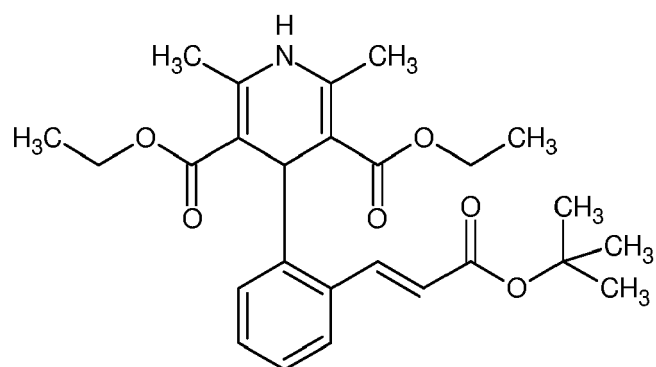
(I-a)
