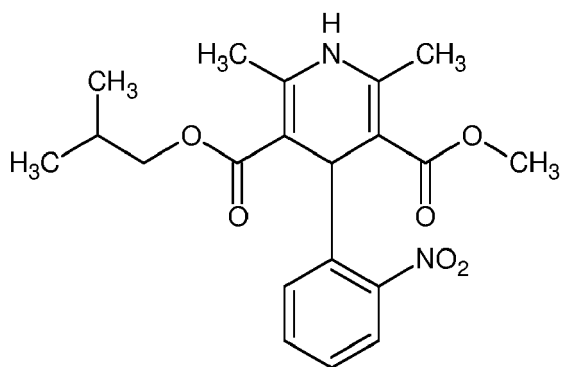
(I-e)
