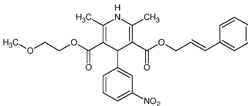
(I-b)
