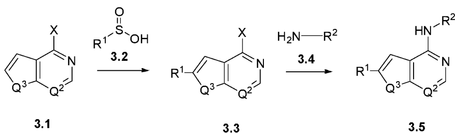
SCHEME 3A.
