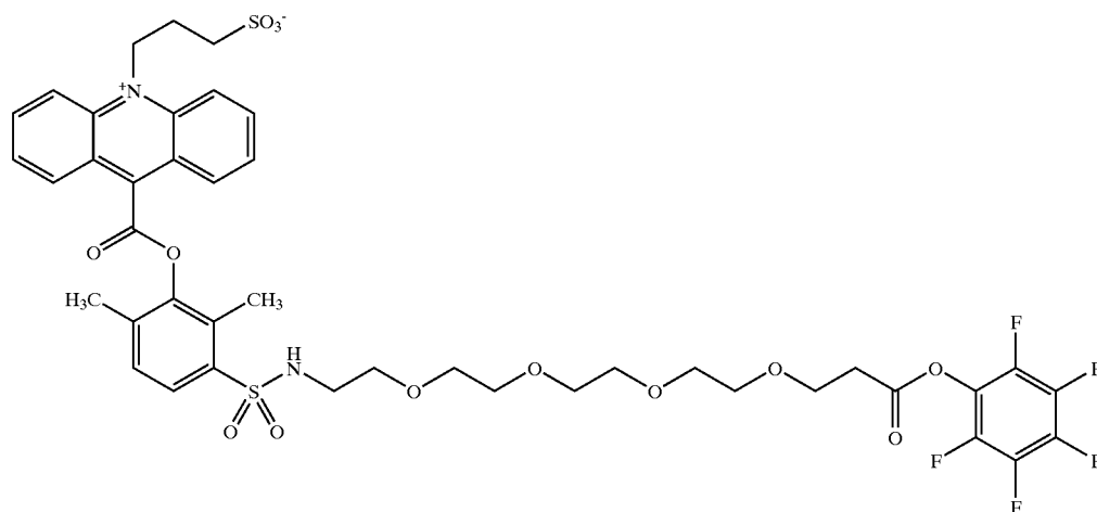
SPAEC-PEO4-PFP
