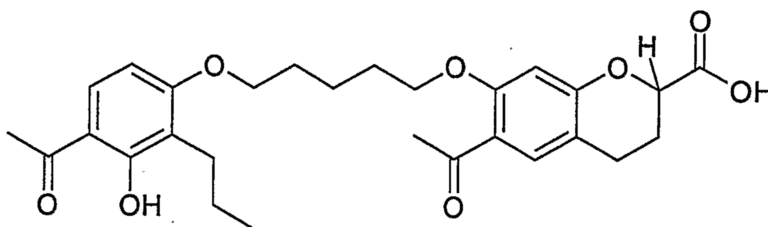
Ablukast
