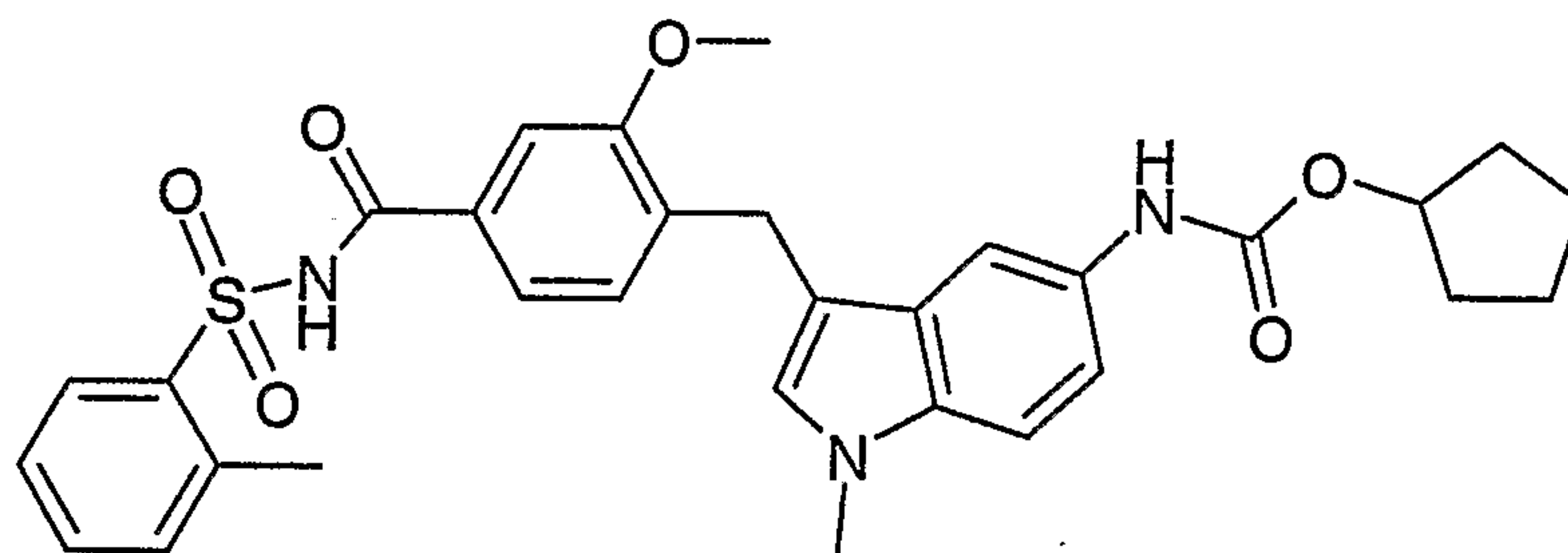
Zafirlukast
