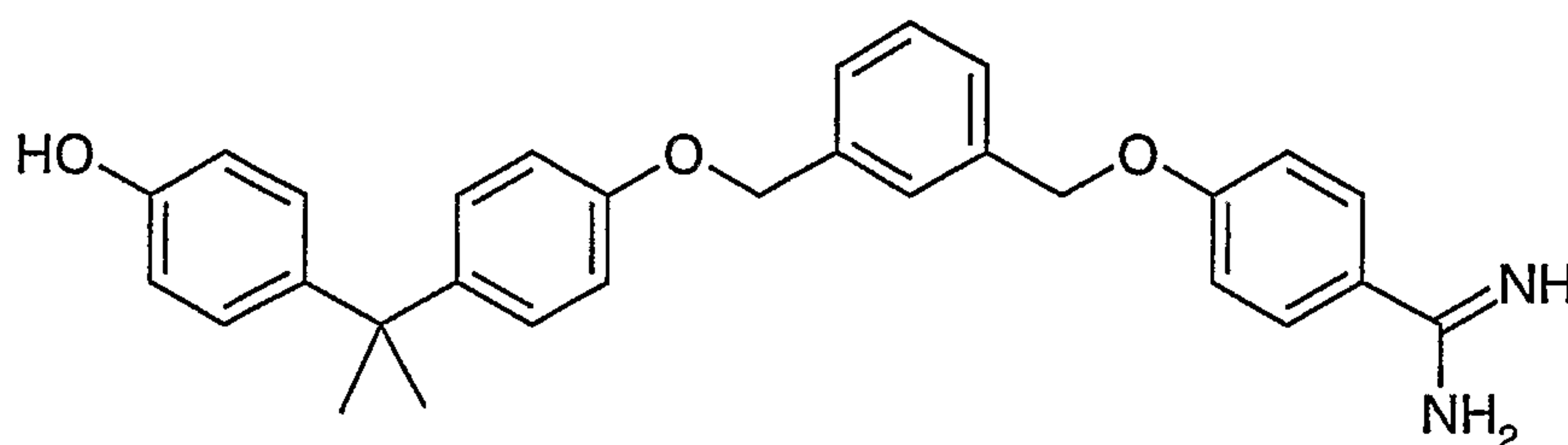
BIIL 284/260
