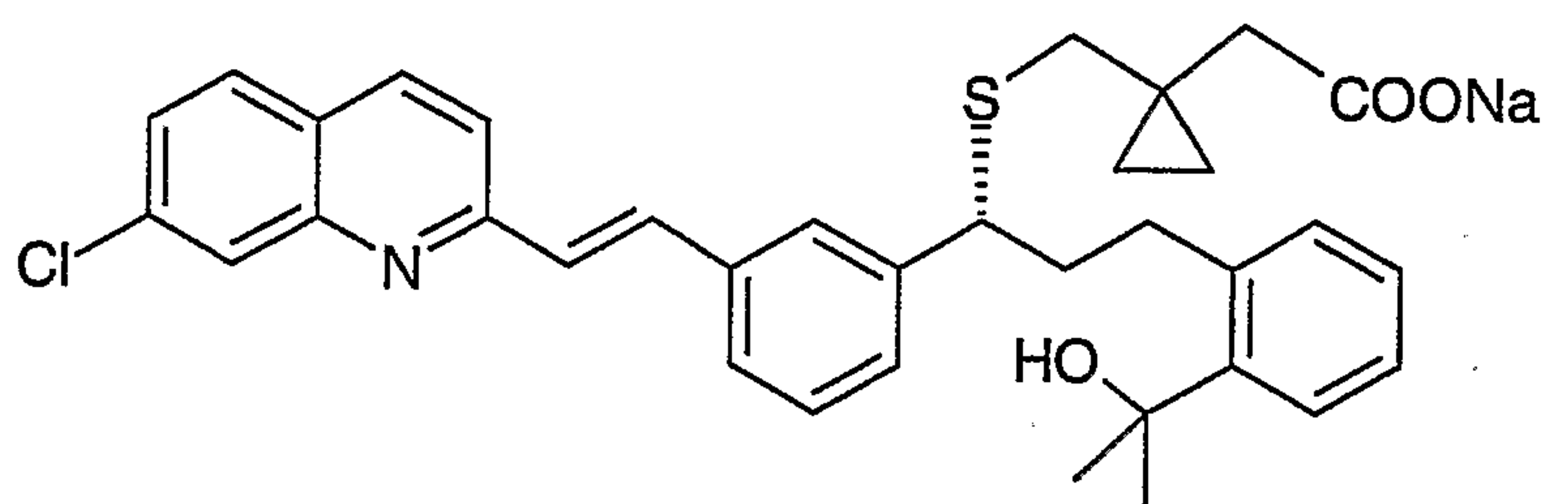
Montekulast
