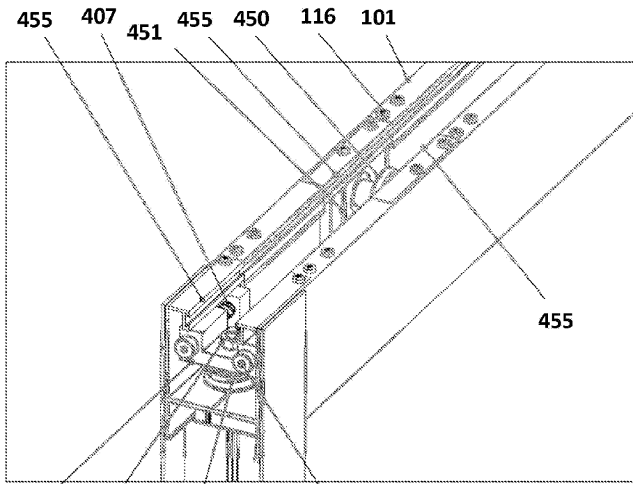
FIG. 26 481 482 402 488
