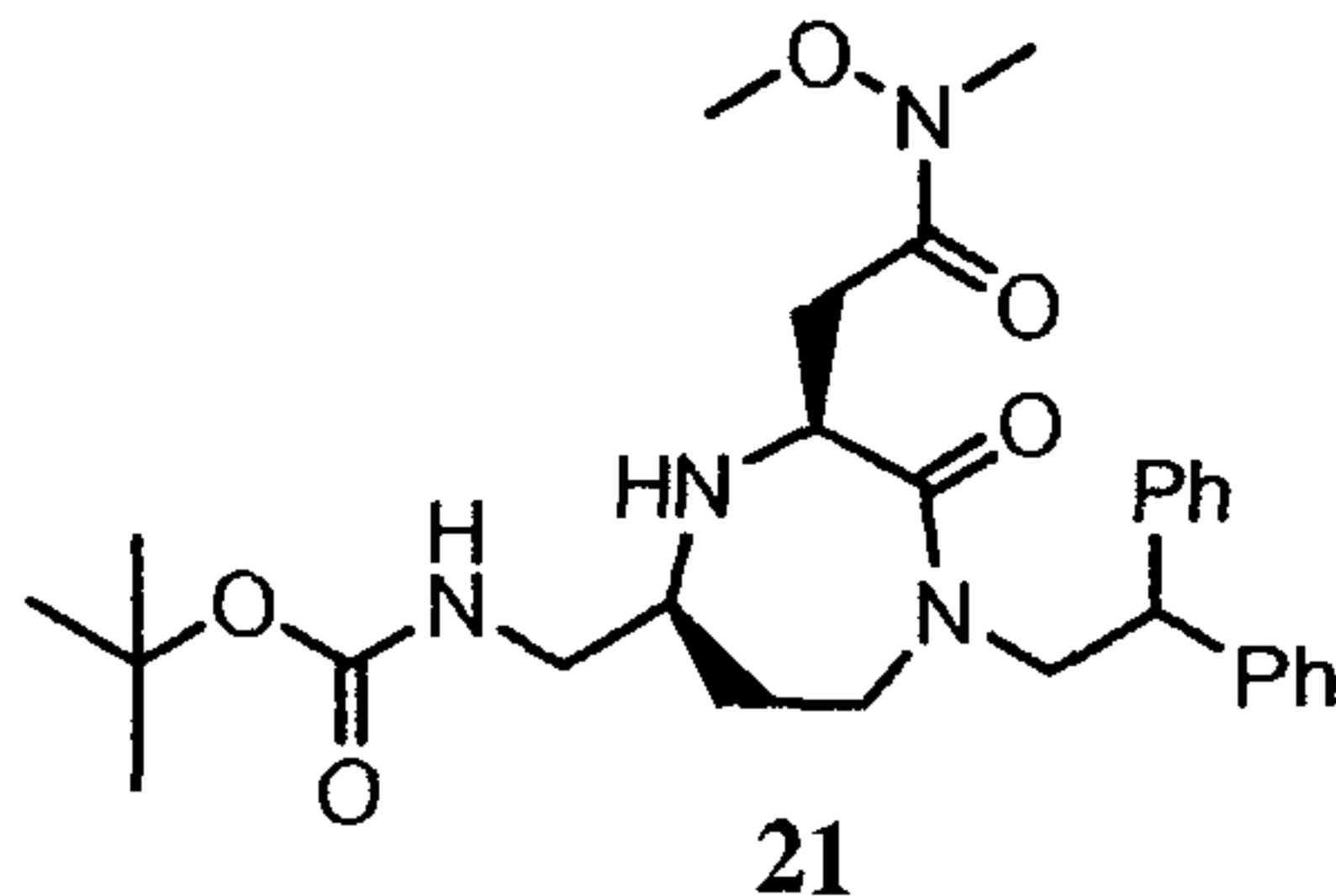
tert-butyl ((3S,5S)-1-(2,2-diphenylethyl)-3-(2-(methoxy(methyl)amino)-2-oxoethyl)-2-oxo-1,4-diazepan-5-yl)methylcarbamate
