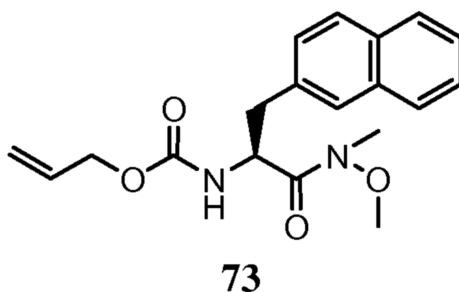
(S)-allyl 1-(methoxy(methyl)amino)-3-(naphthalen-2-yl)-1-oxopropan-2-ylcarbamate
