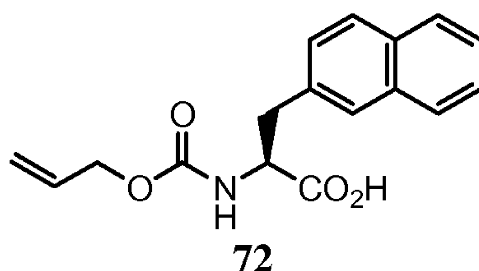
((S)-2-(allyloxycarbonylamino)-3-(naphthalen-2-yl)propanoic acid
