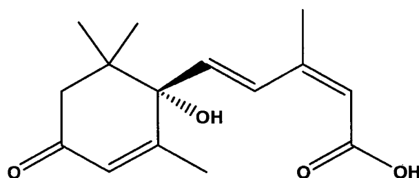
S-Absciscic Acid
