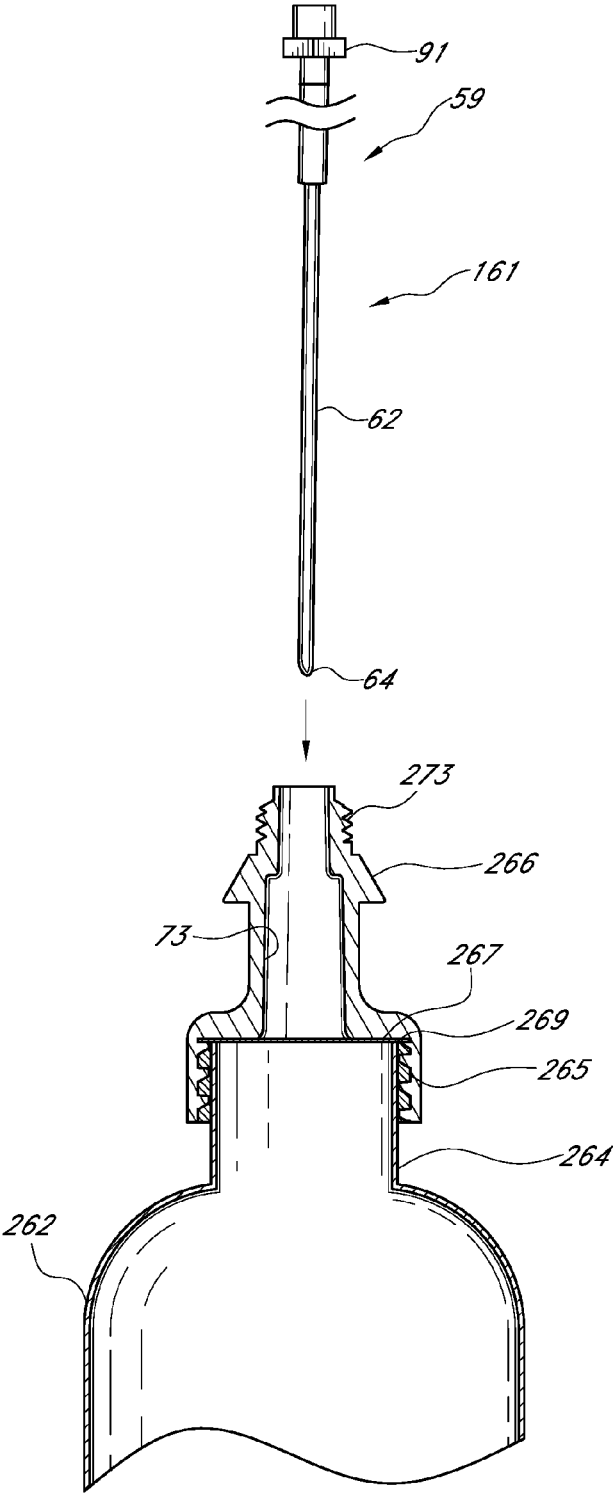
FIG. 13A
