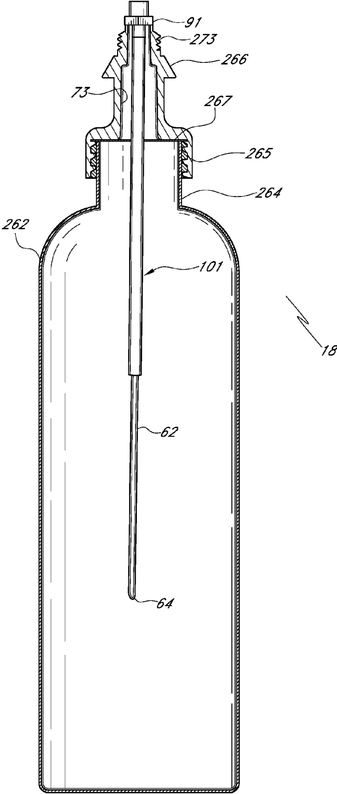
FIG. 13B
