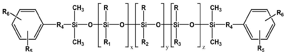
(VII)
