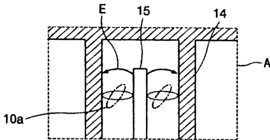
(prior art) FIG. 9A
