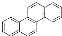
(ae) Chrysene
