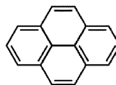
(ag) Pyrene
