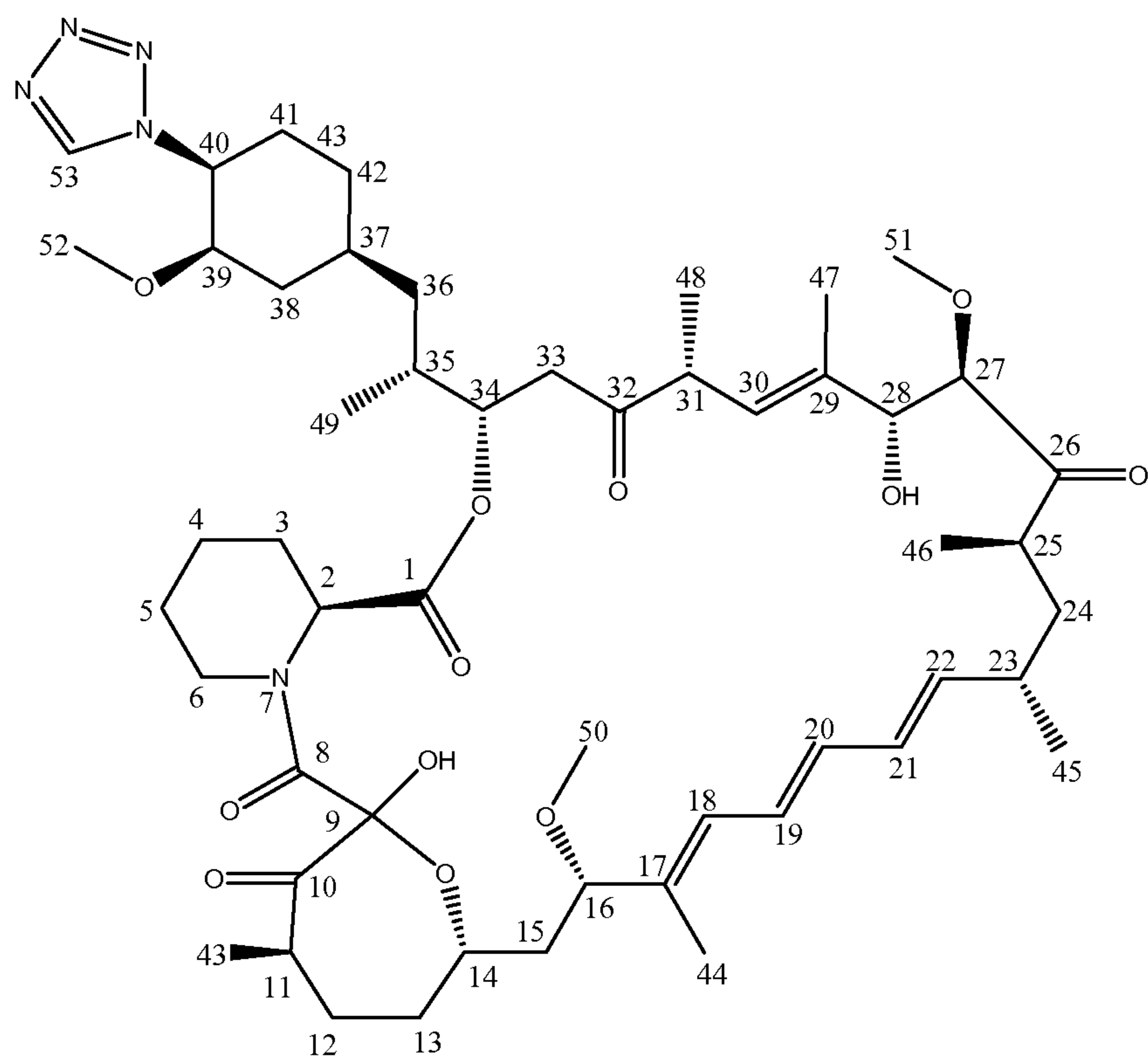
Oxepane 2
