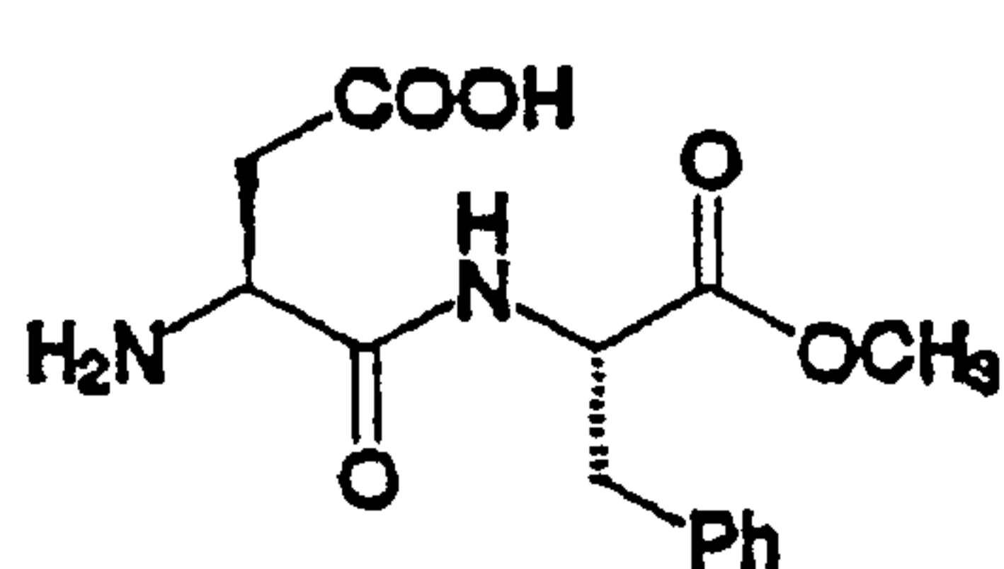
Aspartame
