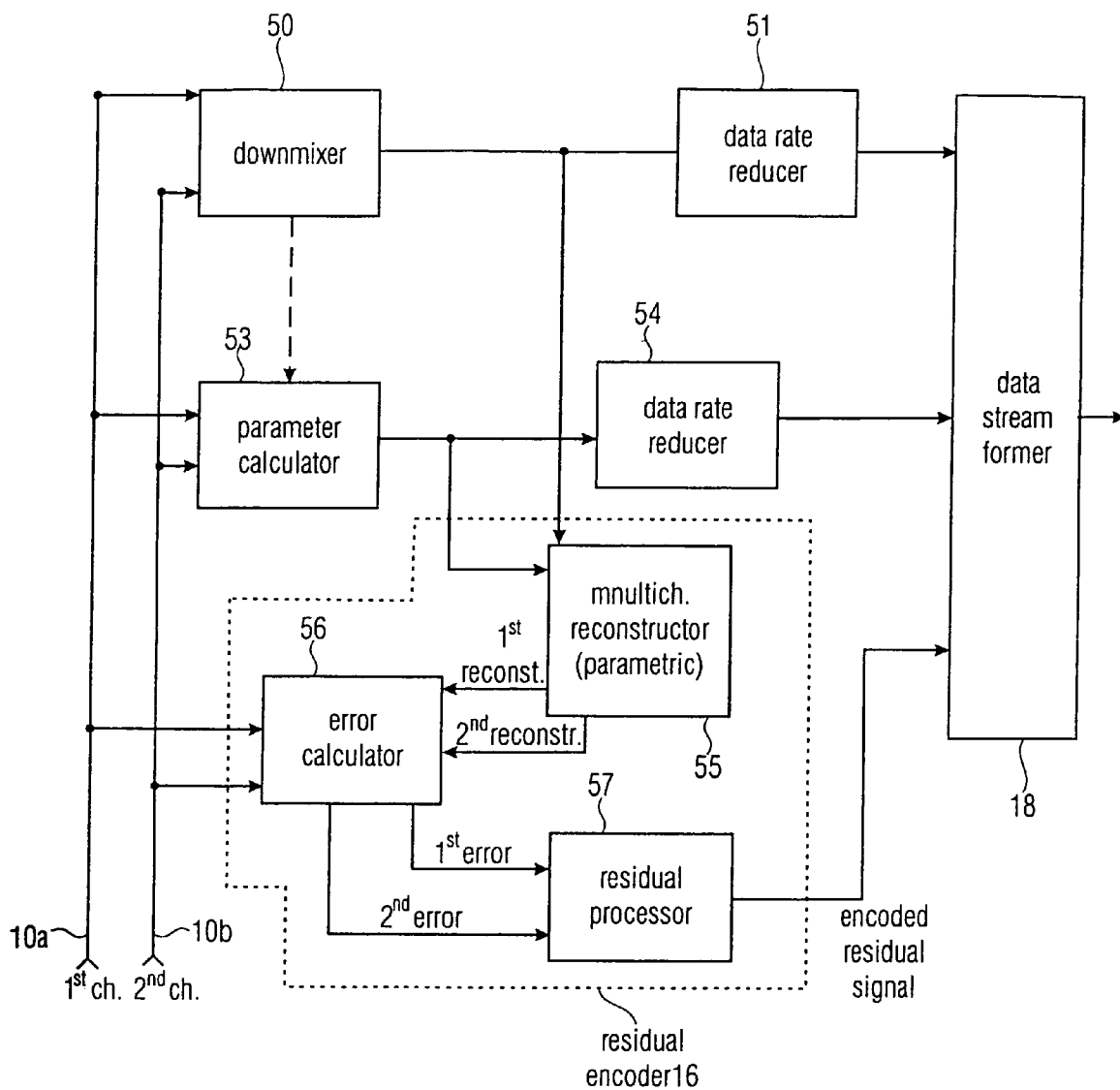
FIG. 5 (Encoder)
