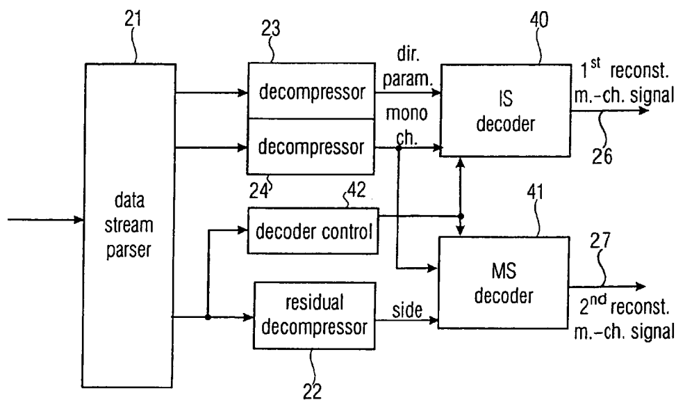
FIG. 4 (Decoder)
