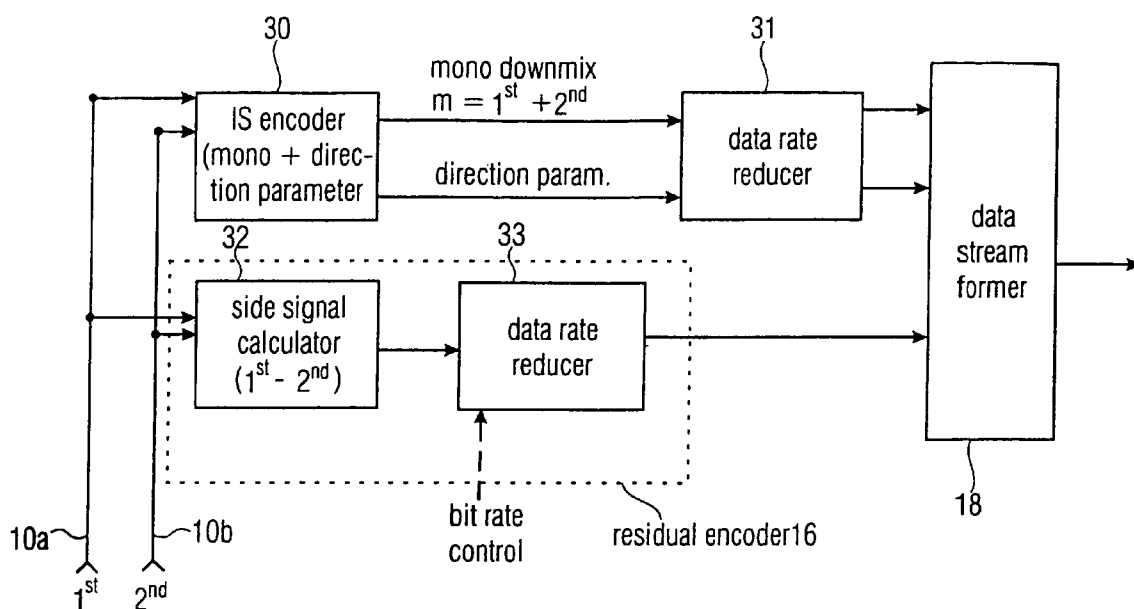
FIG. 3 (Encoder)
