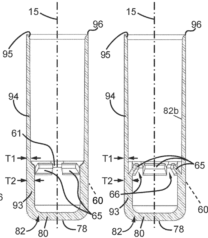
Section C-C FIG. 13C
