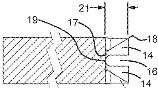
Section A-A FIG. 11
