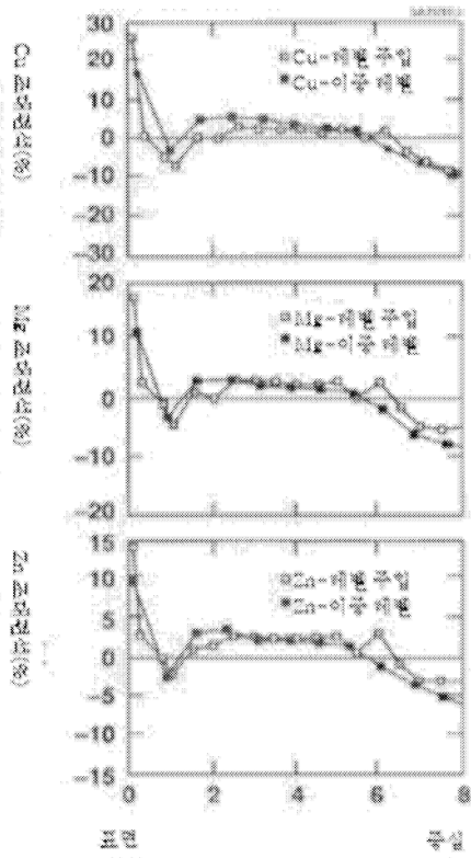
잉곳 표면으로부터의 잉곳 부피에 따른 거리(인치)
