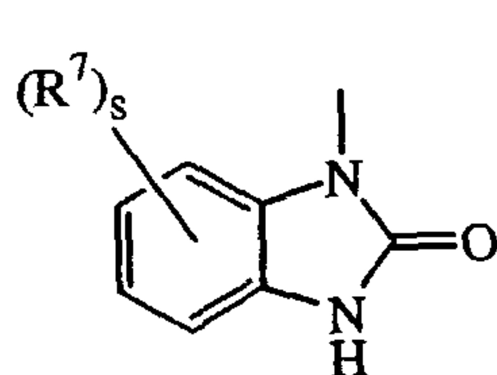
(a-33)
