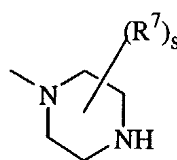
(a-51)
