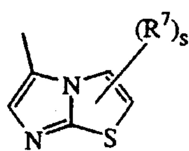
(a-34)
