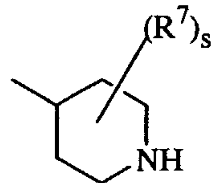
(a-6)
