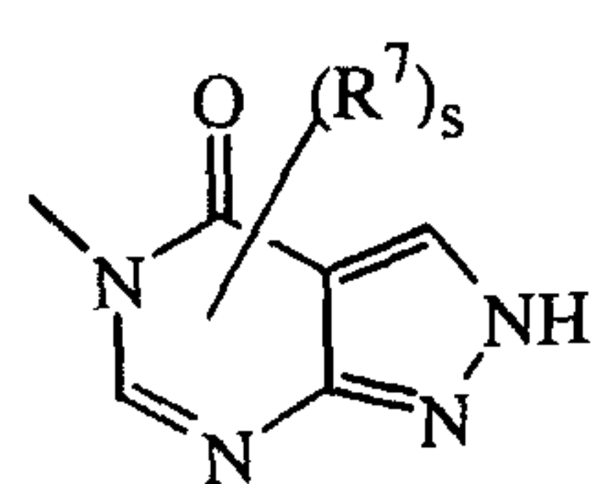
(a-45)
