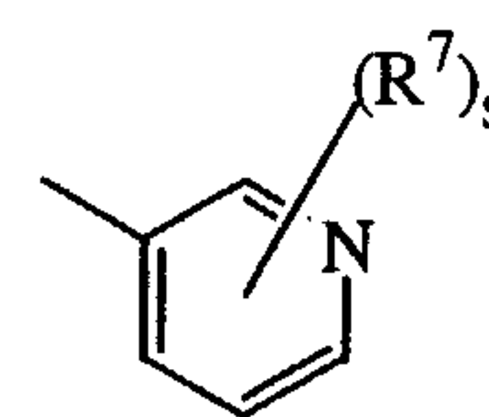
(a-4)
