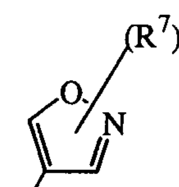
(a-12)
