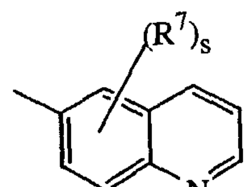
(a-35)
