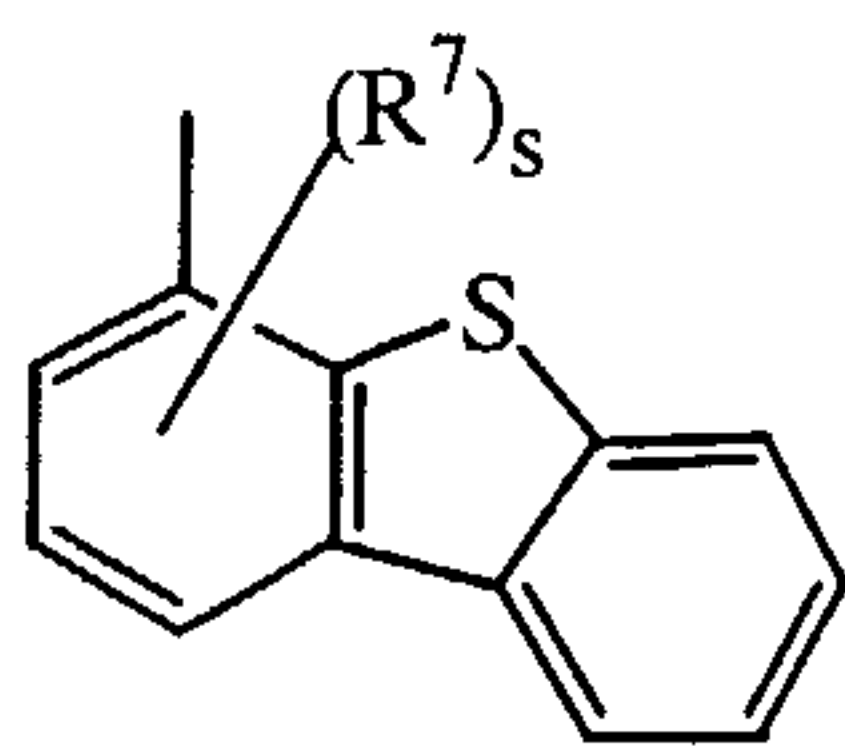
(a-49)
