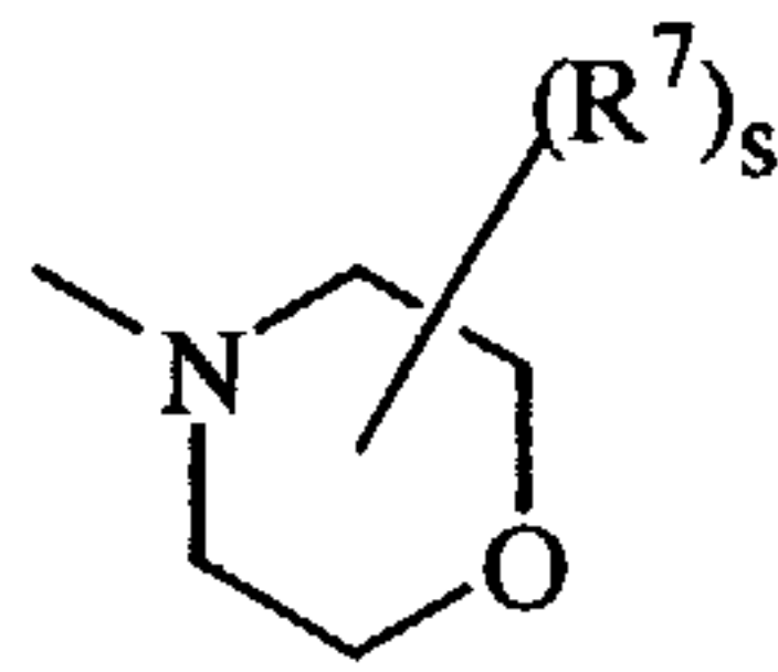
(a-7)
