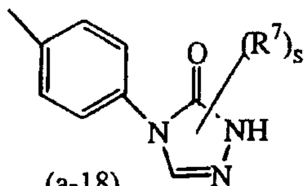
(a-18)
