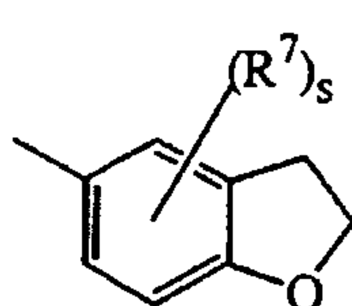
(a-30)
