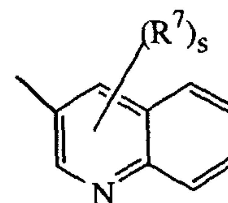
(a-24)
