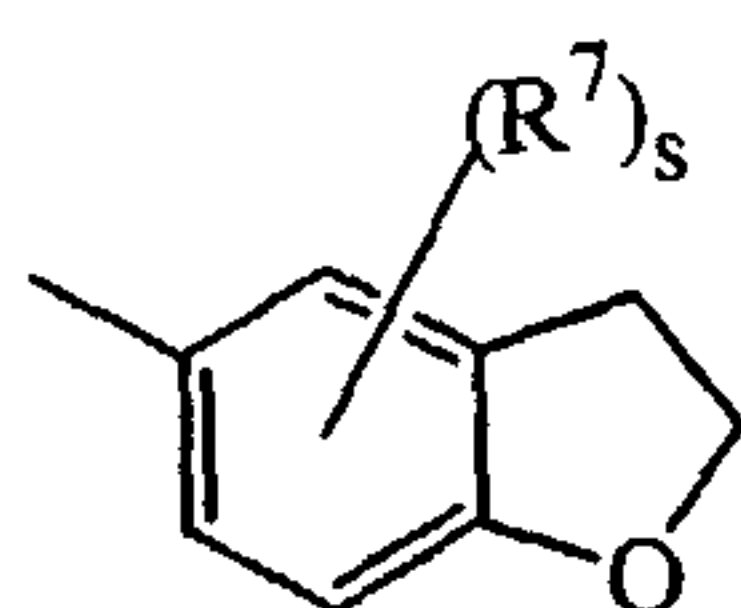
(a-30)
