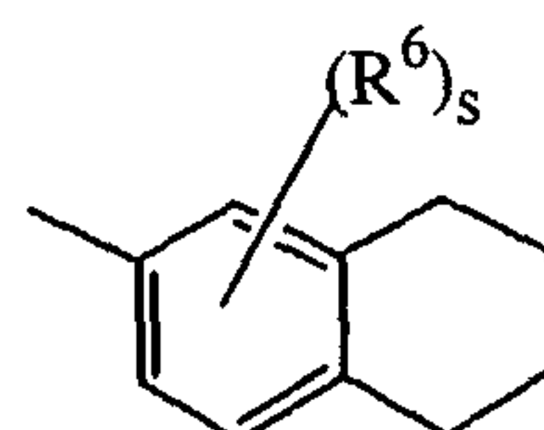
(a-43)
