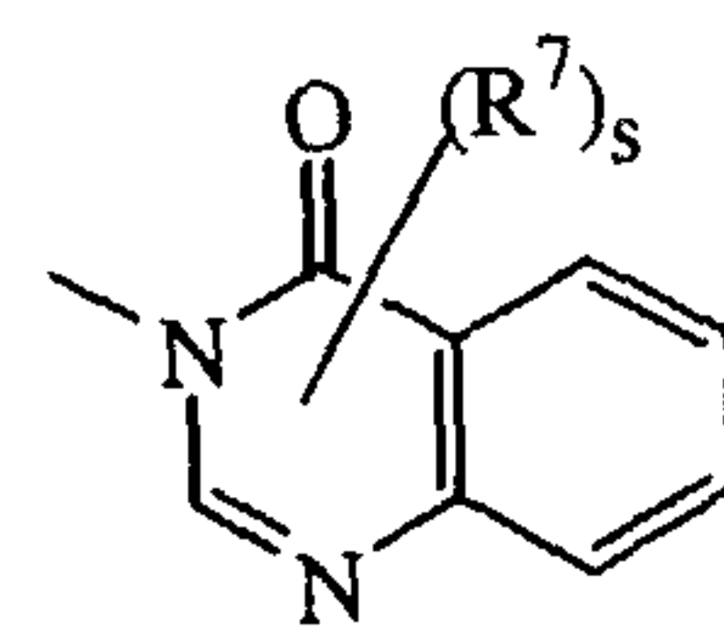
(a-47)
