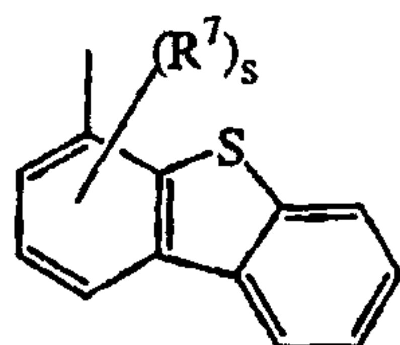
(a-49)
