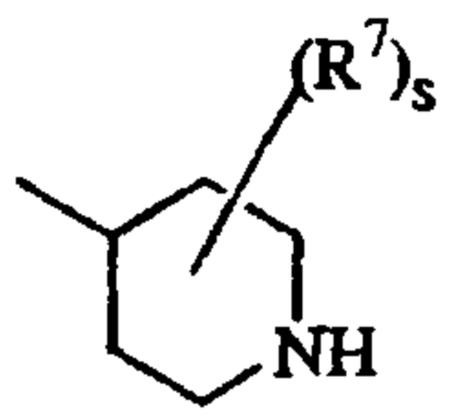
(a-6)
