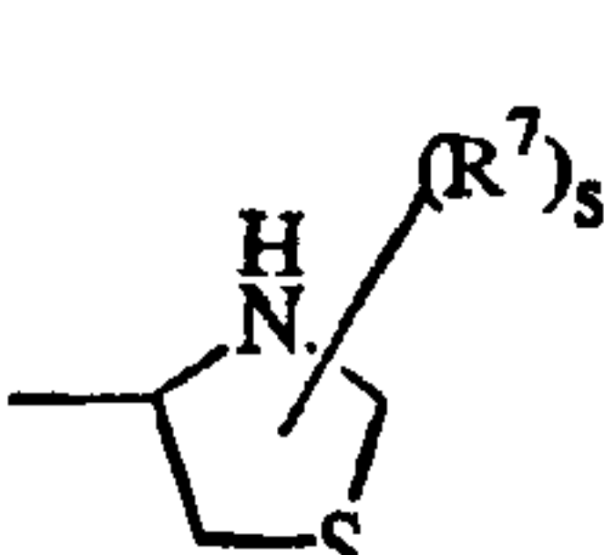
(a-16)
