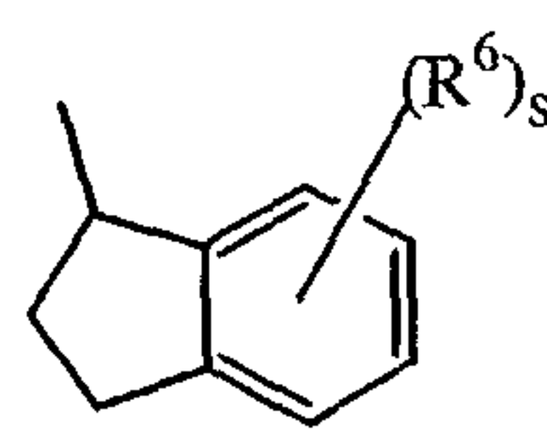
(a-27)
