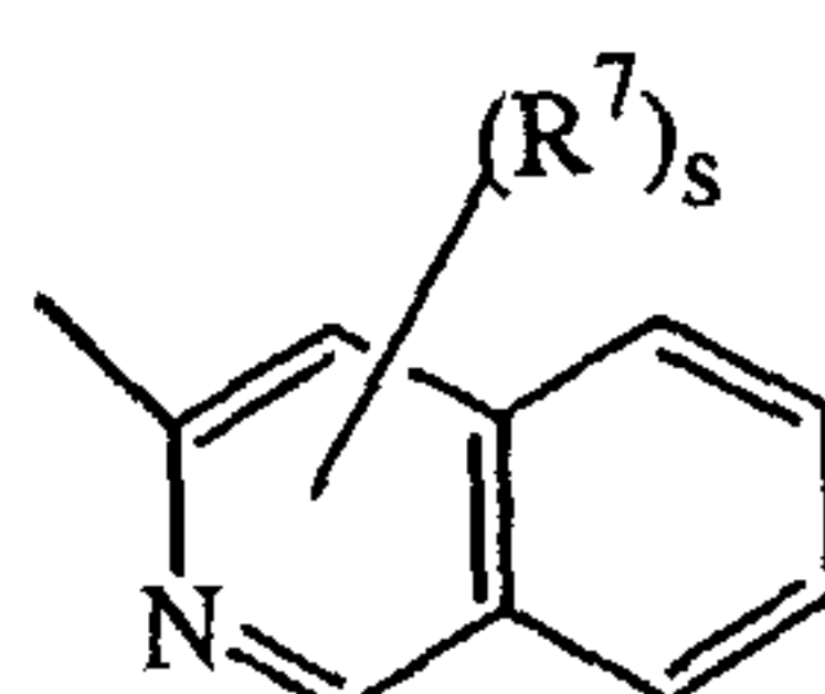
(a-42)
