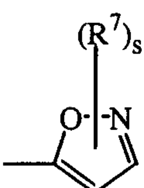
(a-13)
