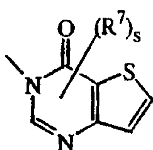
(a-46)
