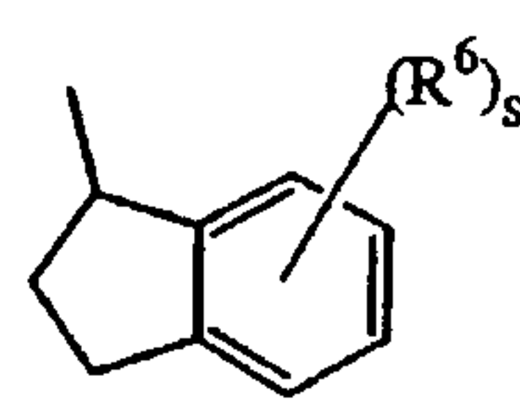
(a-27)
