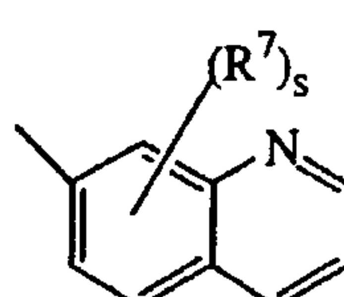
(a-23)
