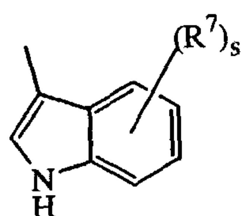
(a-29)
