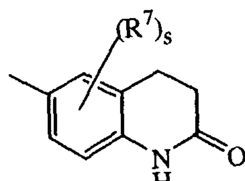
(a-38)
