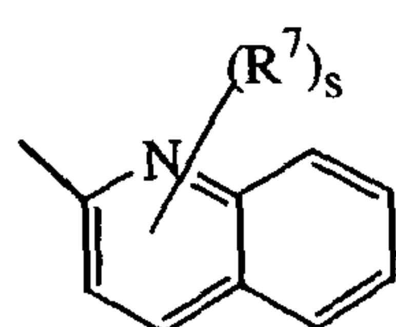
(a-41)
