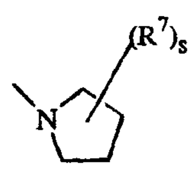
(a-44)
