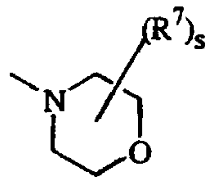
(a-7)
