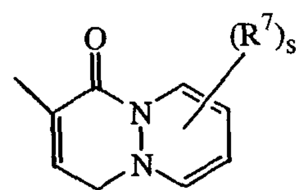
(a-35)
