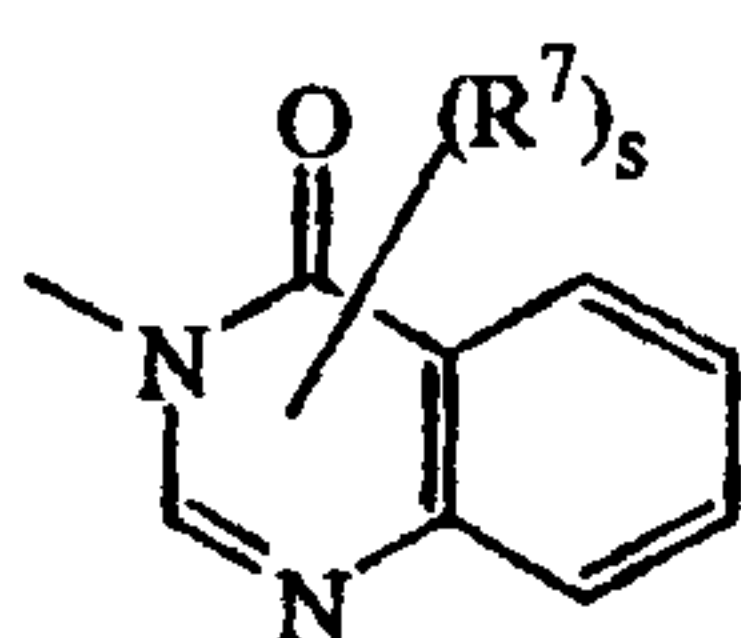
(a-47)
