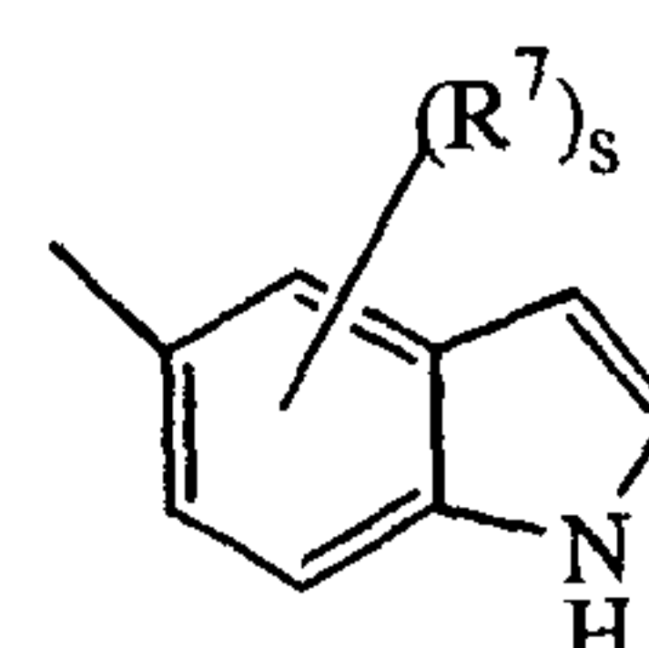
(a-48)
