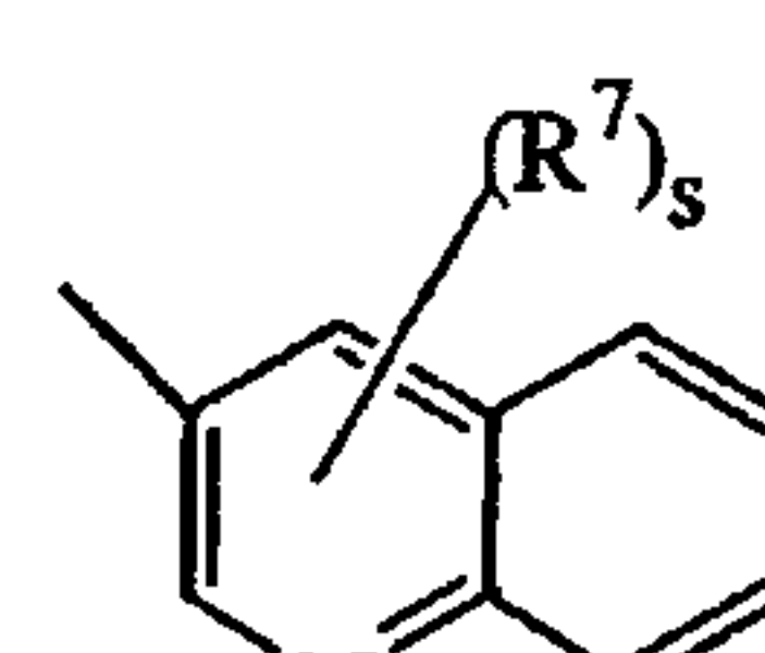
(a-24)
