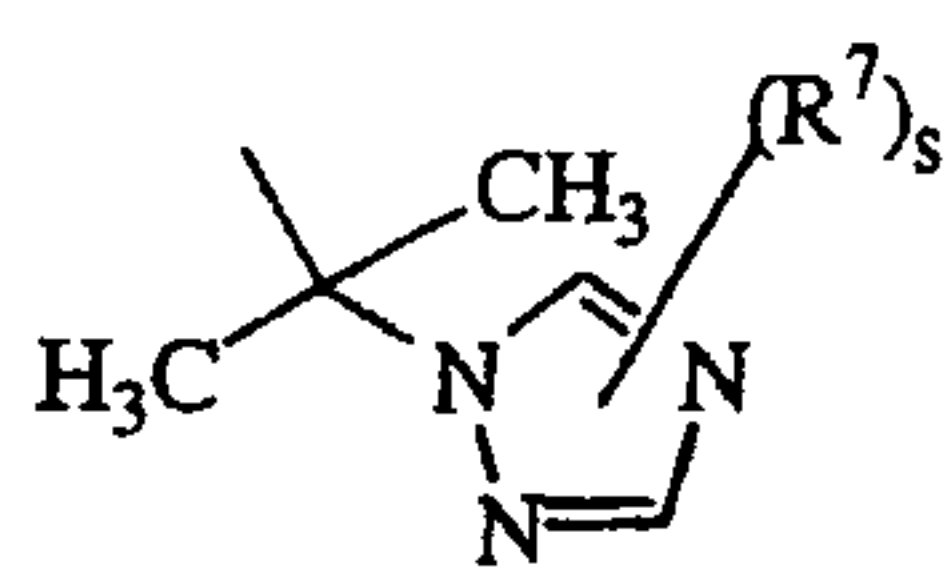
(a-17)
