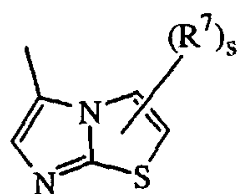
(a-34)
