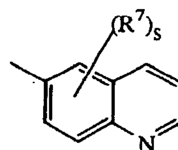
(a-39)
