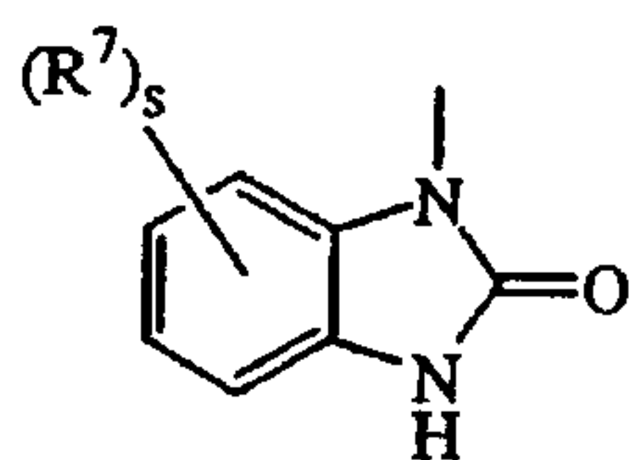
(a-33)
