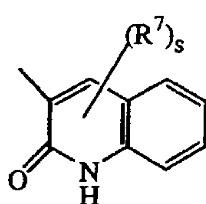
(a-26)
