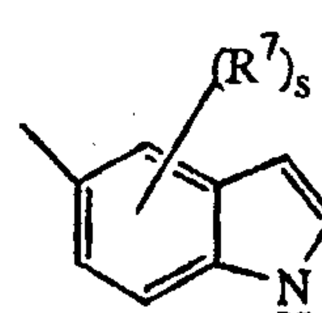
(a-48)
