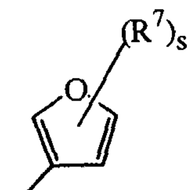
(a-40)
