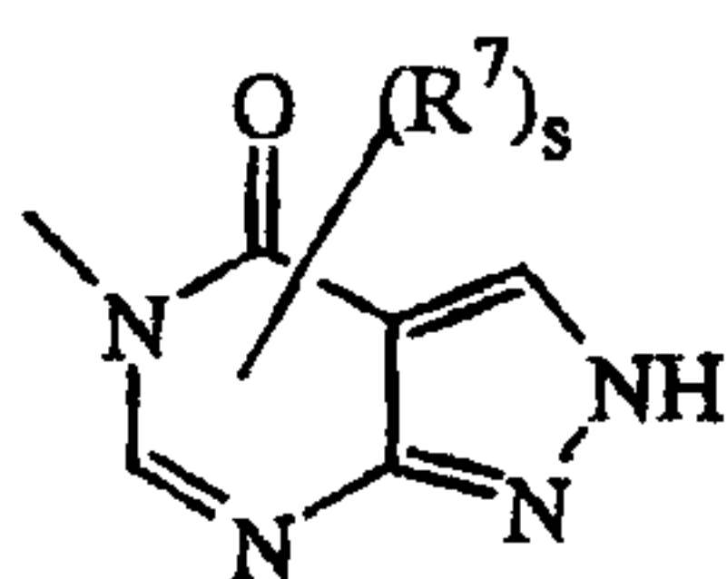
(a-45)
