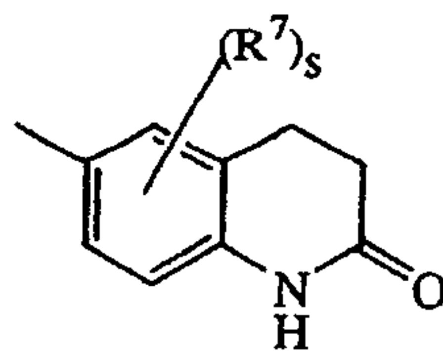
(a-38)
