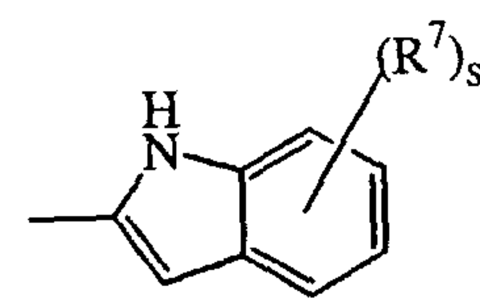
(a-28)
