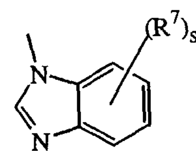
(a-36)
