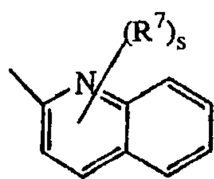
(a-41)
