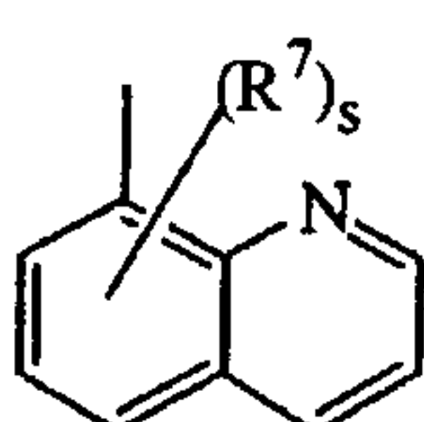
(a-22)
