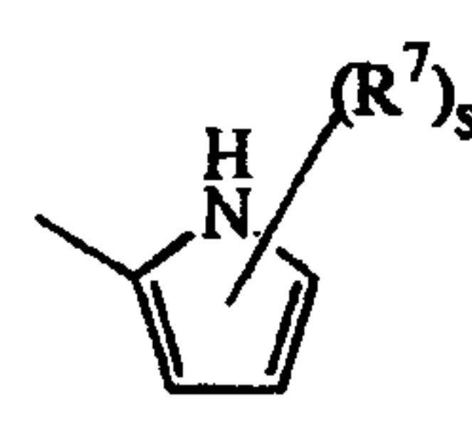
(a-8)
