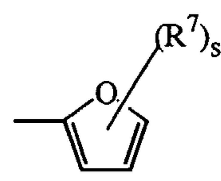
(a-11)
