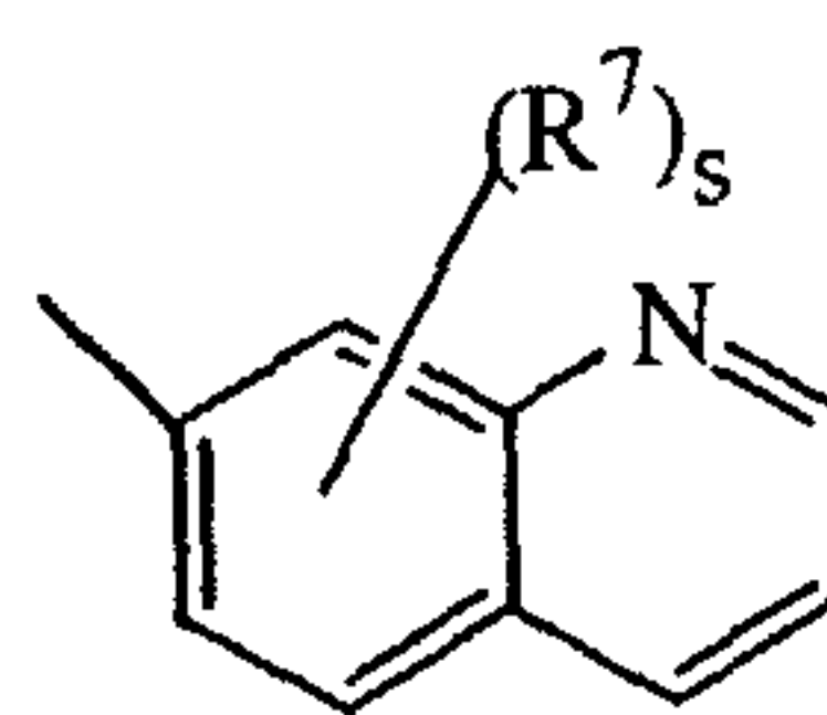
(a-23)
