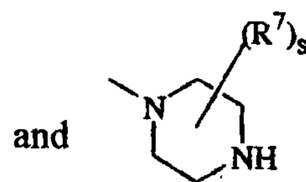
(a-51) ,
