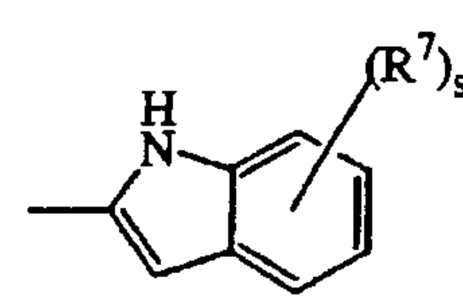
(a-28)
