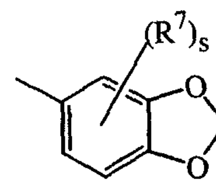
(a-32)
