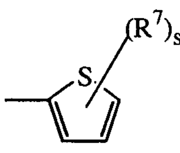
(a-9)
