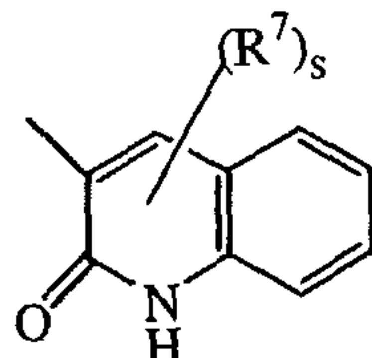
(a-26)
