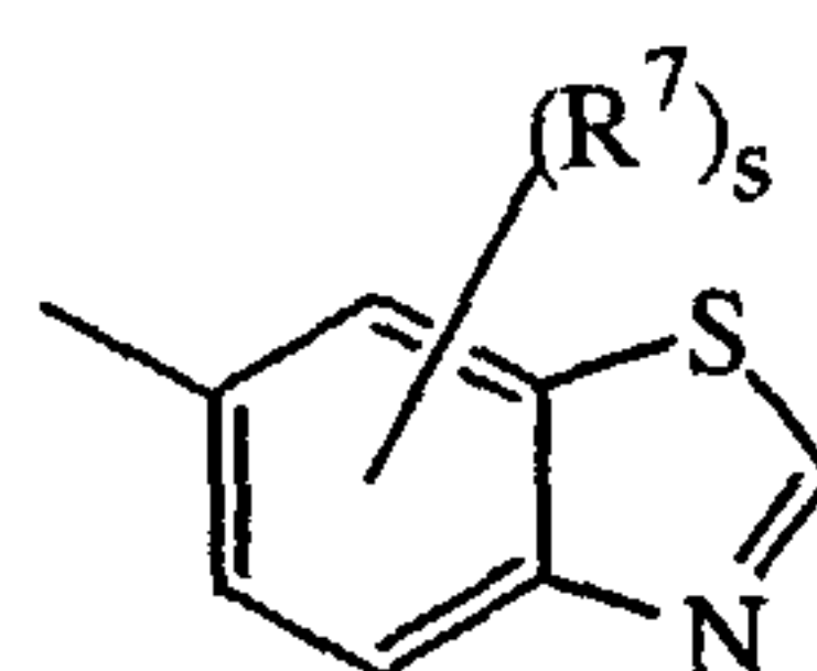
(a-31)
