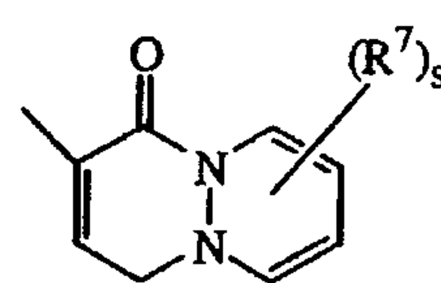
(a-35)
