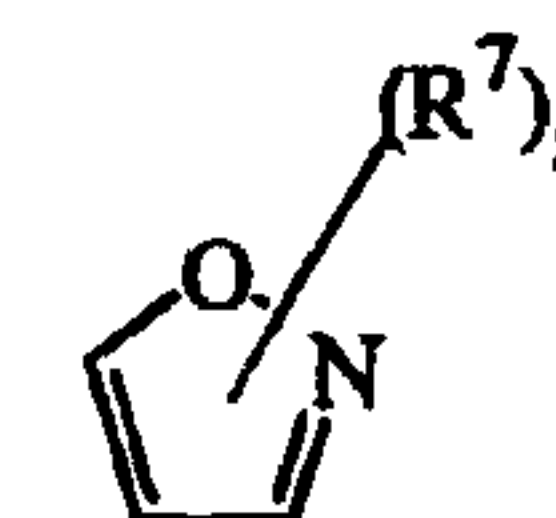
(a-12)
