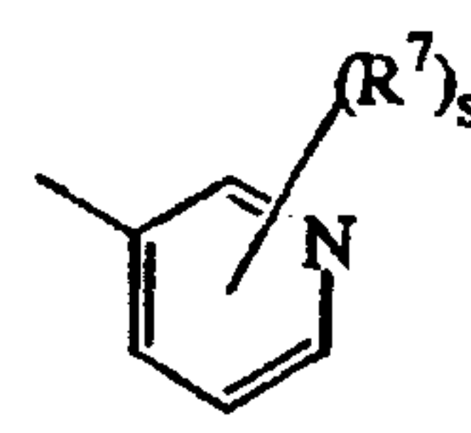
(a-4)
