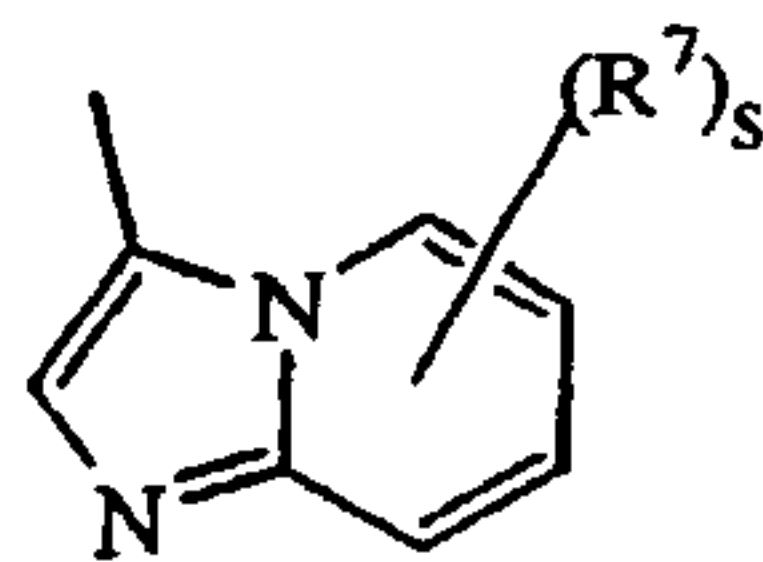
(a-33)
