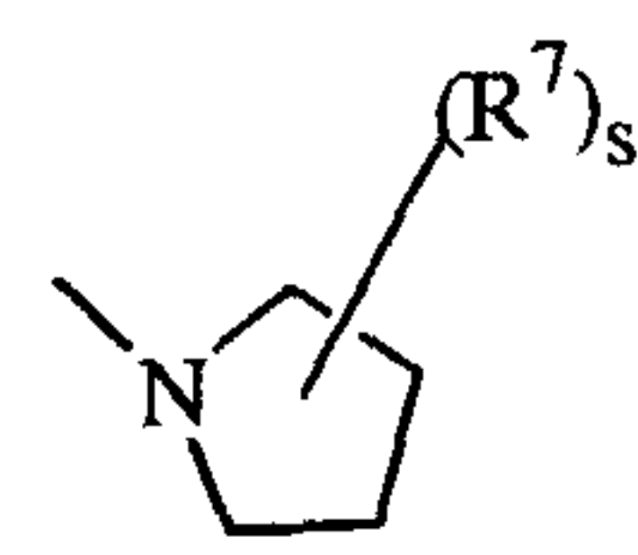
(a-44)
