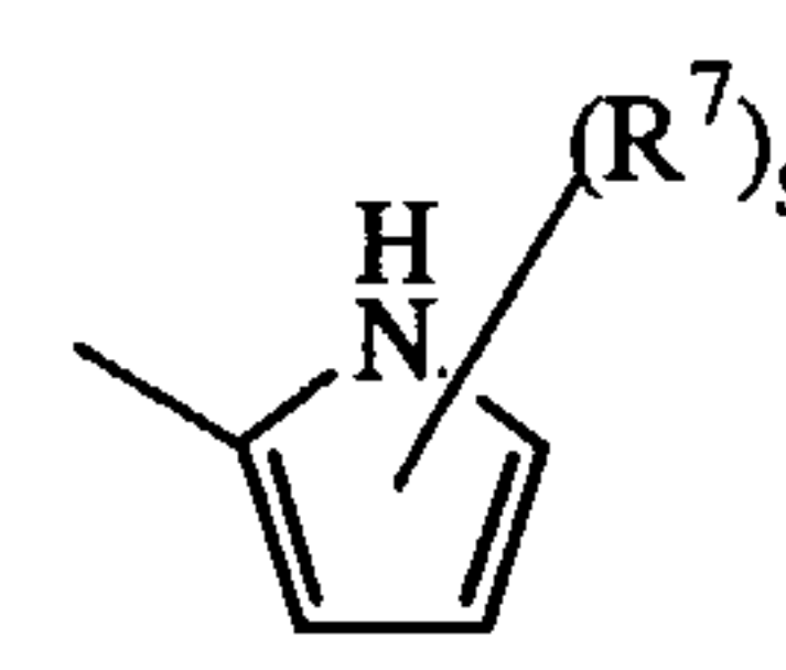
(a-8)
