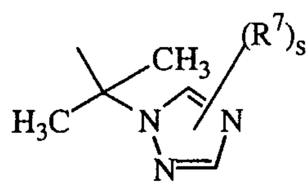
(a-17)
