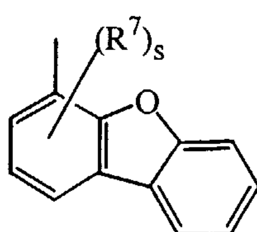
(a-50)
