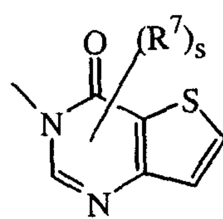
(a-46)
