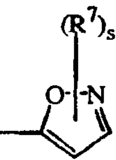
(a-13)
