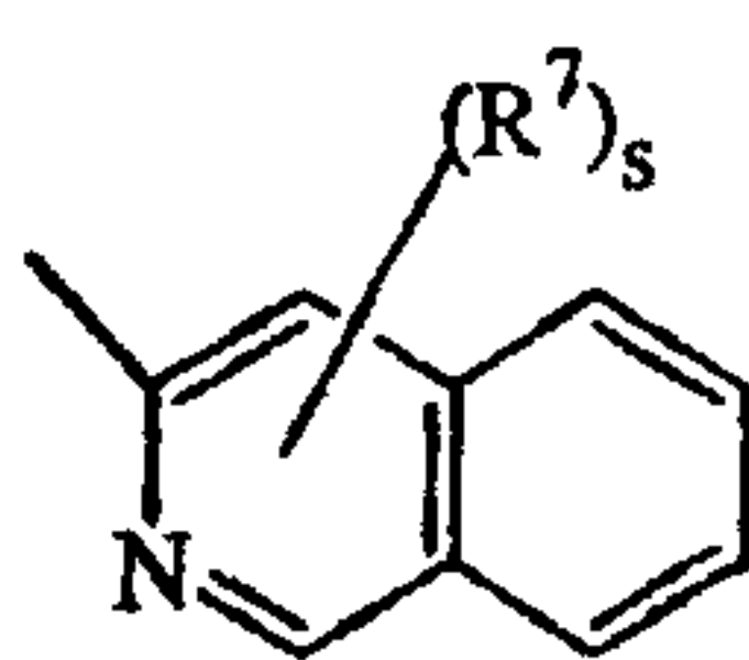
(a-42)
