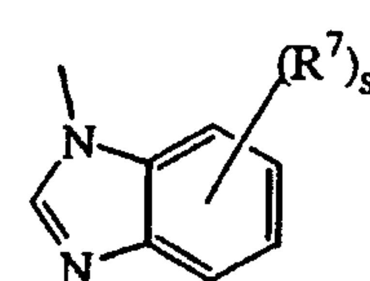
(a-36)
