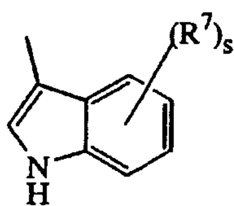
(a-29)
