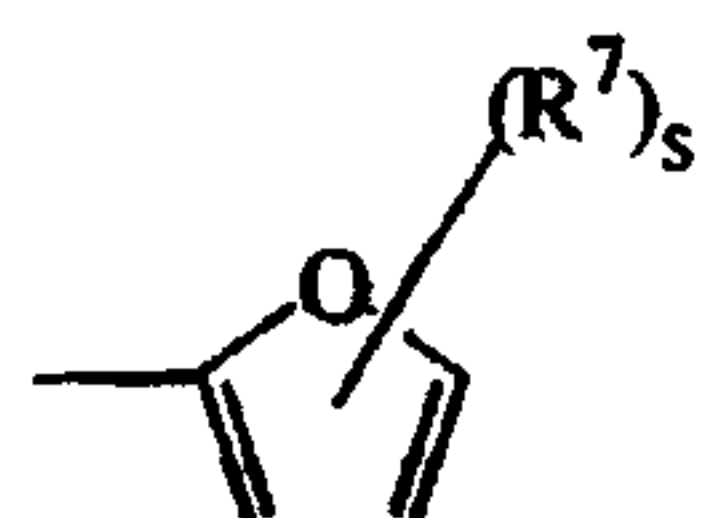
(a-11)
