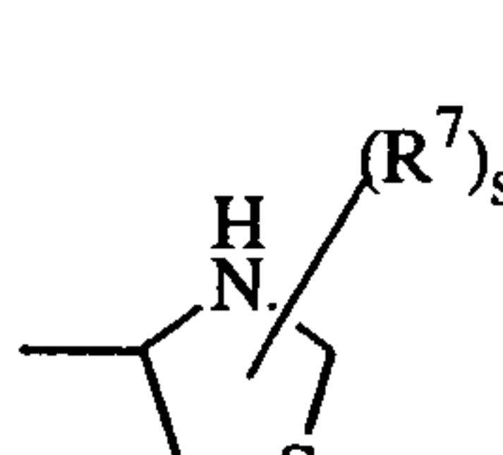
(a-16)
