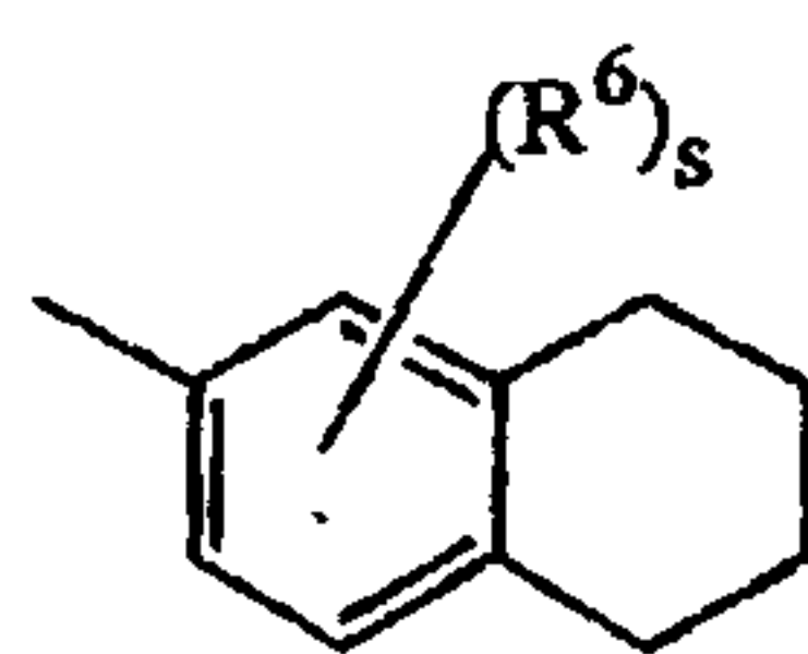
(a-43)
