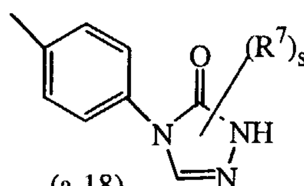
(a-18)
