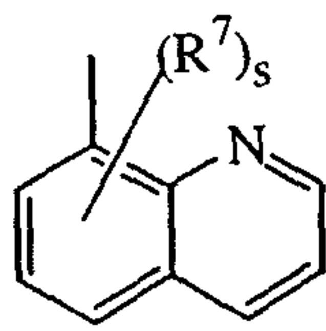
(a-22)
