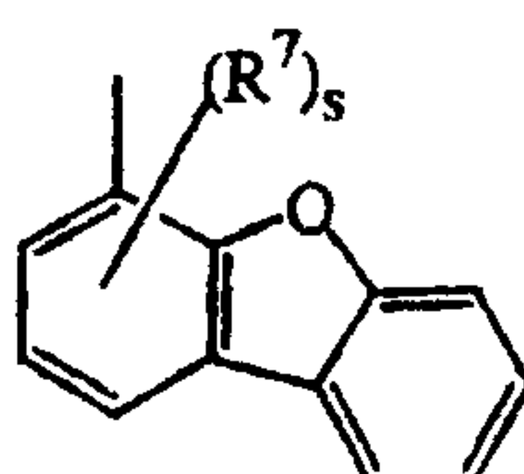
(a-50)
