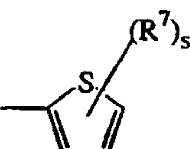
(a-9)
