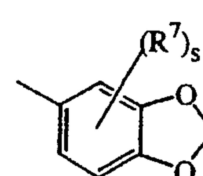
(a-32)
