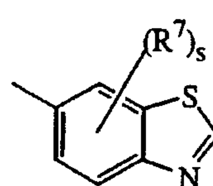
(a-31)
