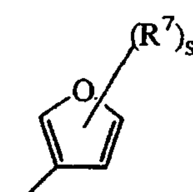
(a-40)
