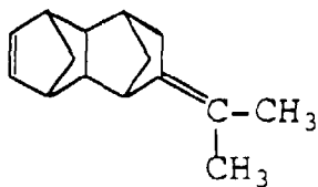
(446) 8-isopropylidene-9-methyltetracyclo[4.4.0.12.5.17,10]-3-dodecene
