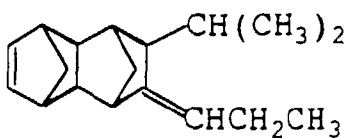
(444) 8-n-propylidene-9-butyltetracyclo[4.4.0.12.5.17,10]-3-dodecene
