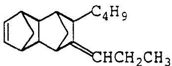
(445) 8-isopropylidenetetracyclo[4.4.0.12.5.17,10]-3-dodecene
