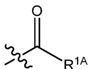
L^1
