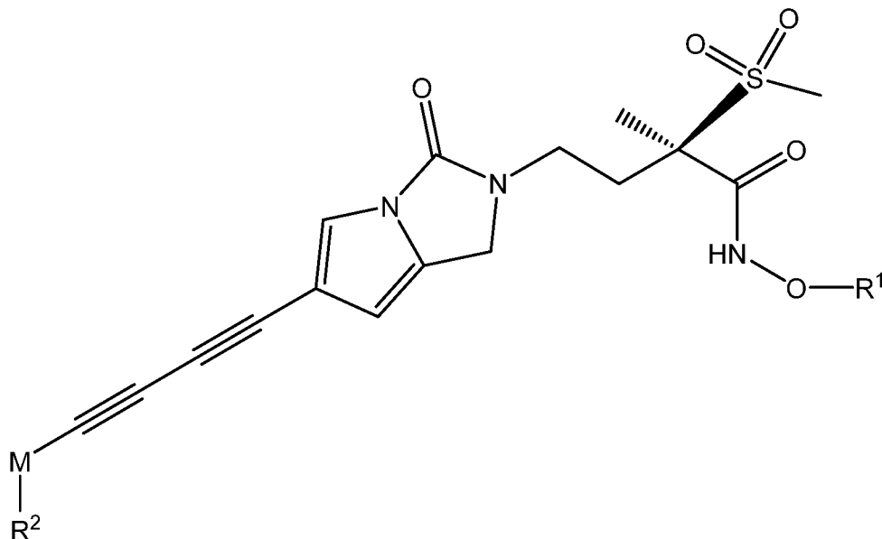
I_{CE}
