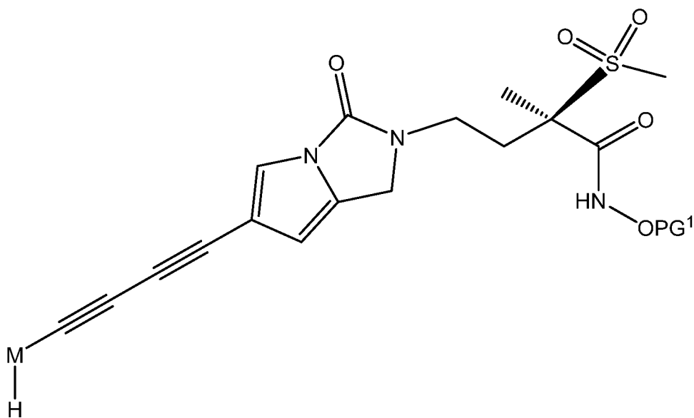
VII
