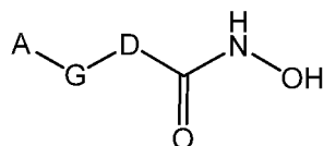
(A0)
