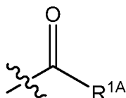
L^1
