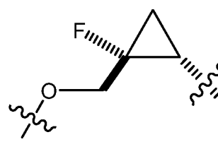
M^C
