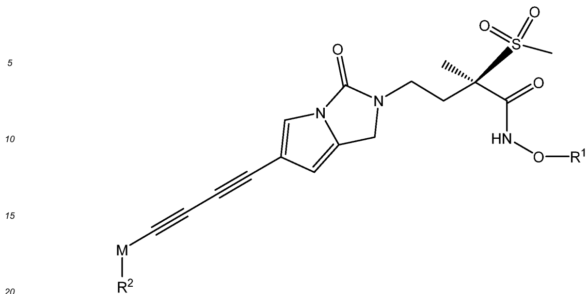
I CE
