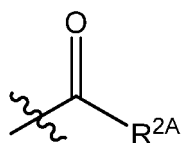
L^{2A}
