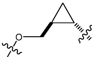
M^B
