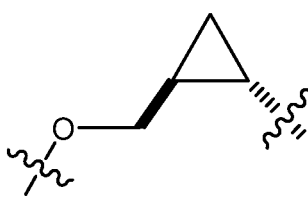
M^B
