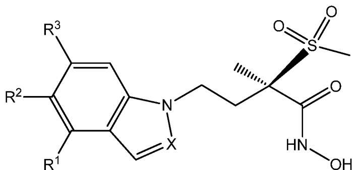
(A2)
