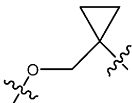
M^A
