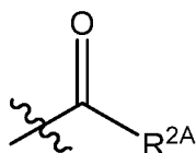
L^{2A}
