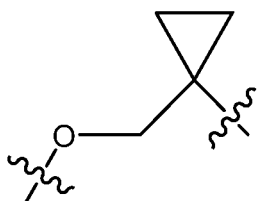
M^A
