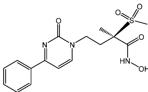
(A6)
