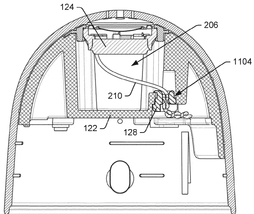
Section D-D
