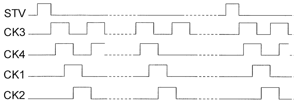
FIG. 14A
