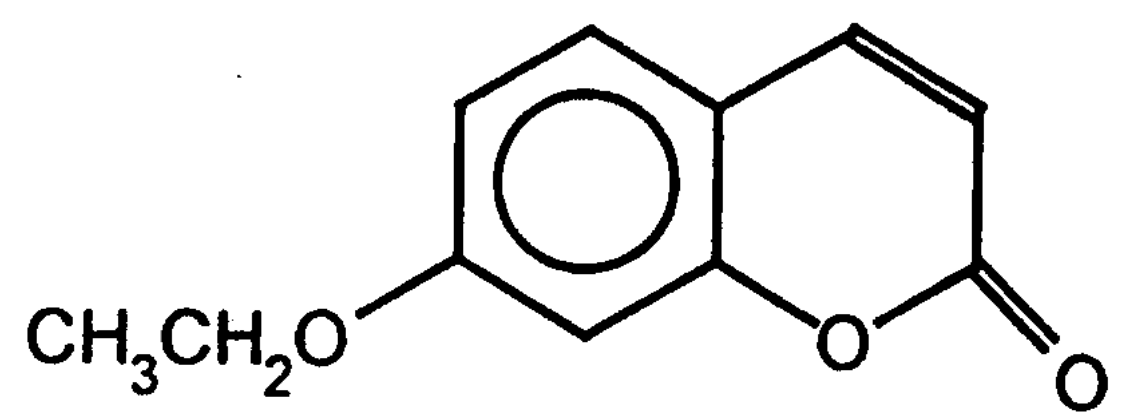
7-Ethoxycoumarin
