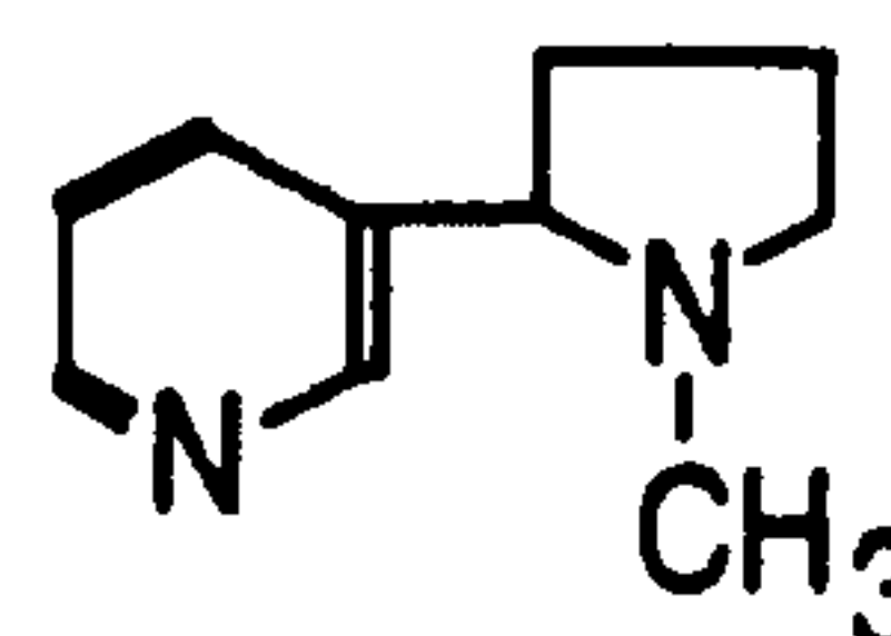
Nicotine
