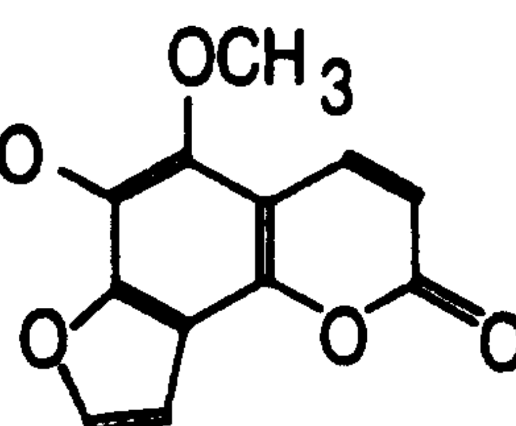
Pimpinlin IC 50 >500
