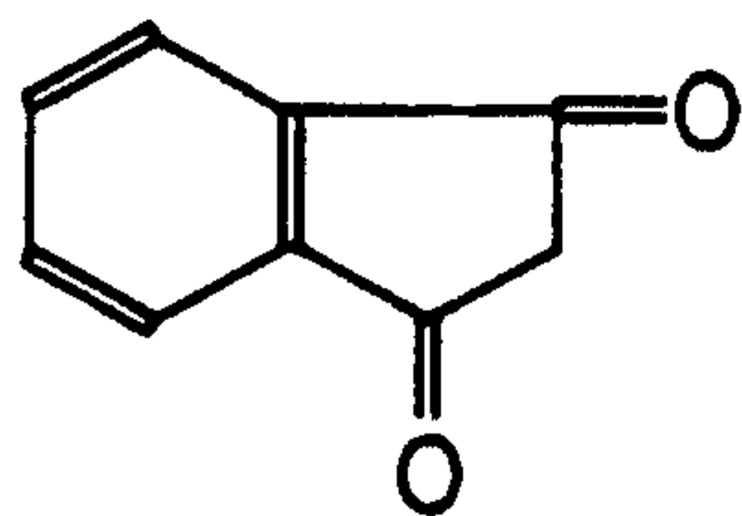
1,3-Indandione
