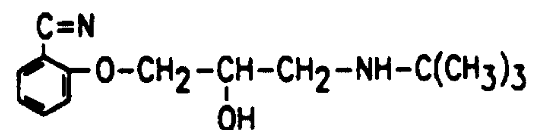
Bunitrolo
