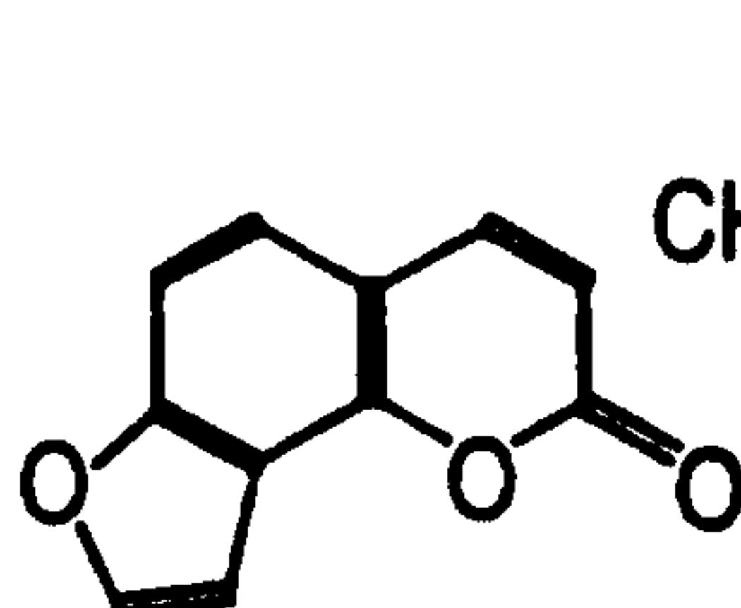
Amgelicin IC 50 160
