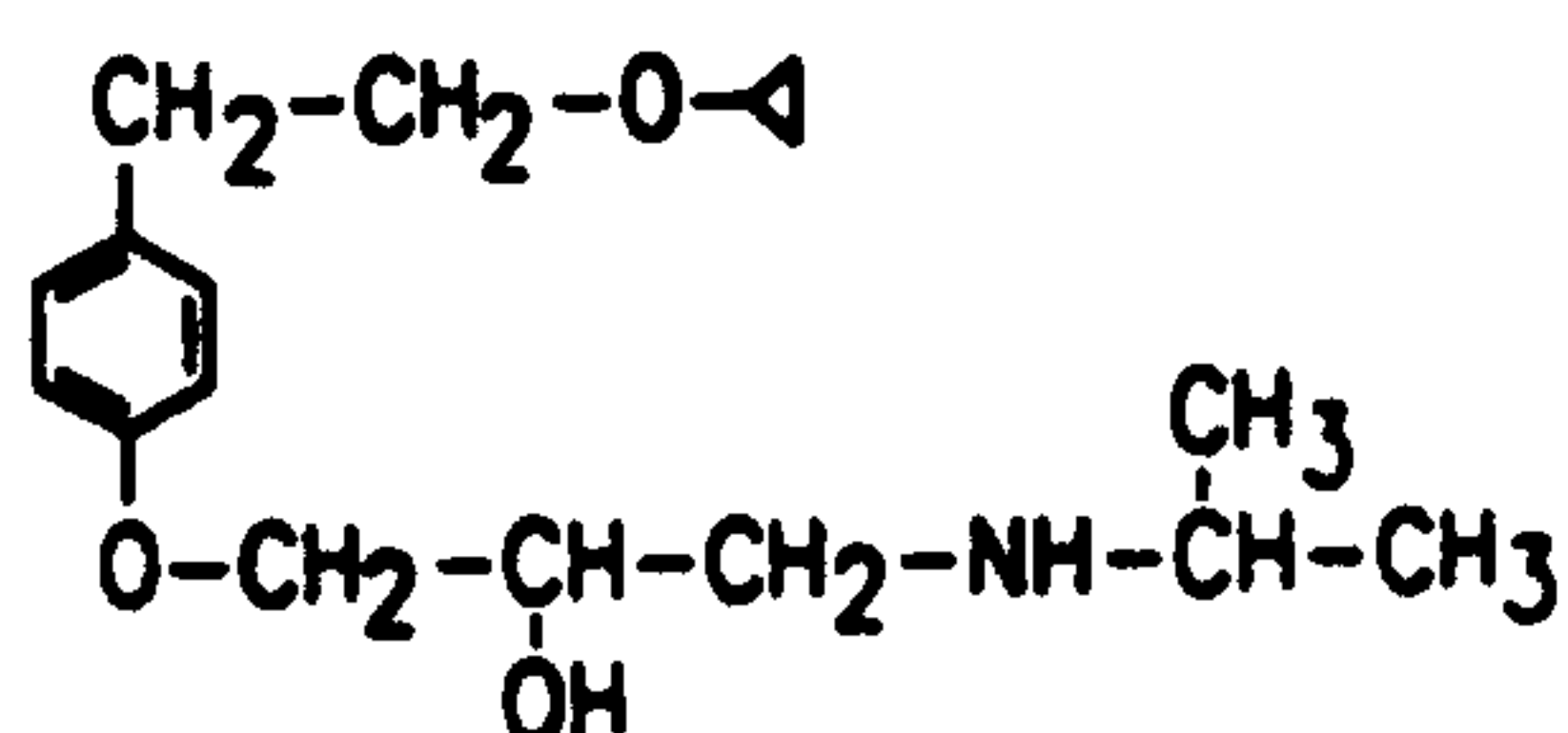
Betaxoiol
