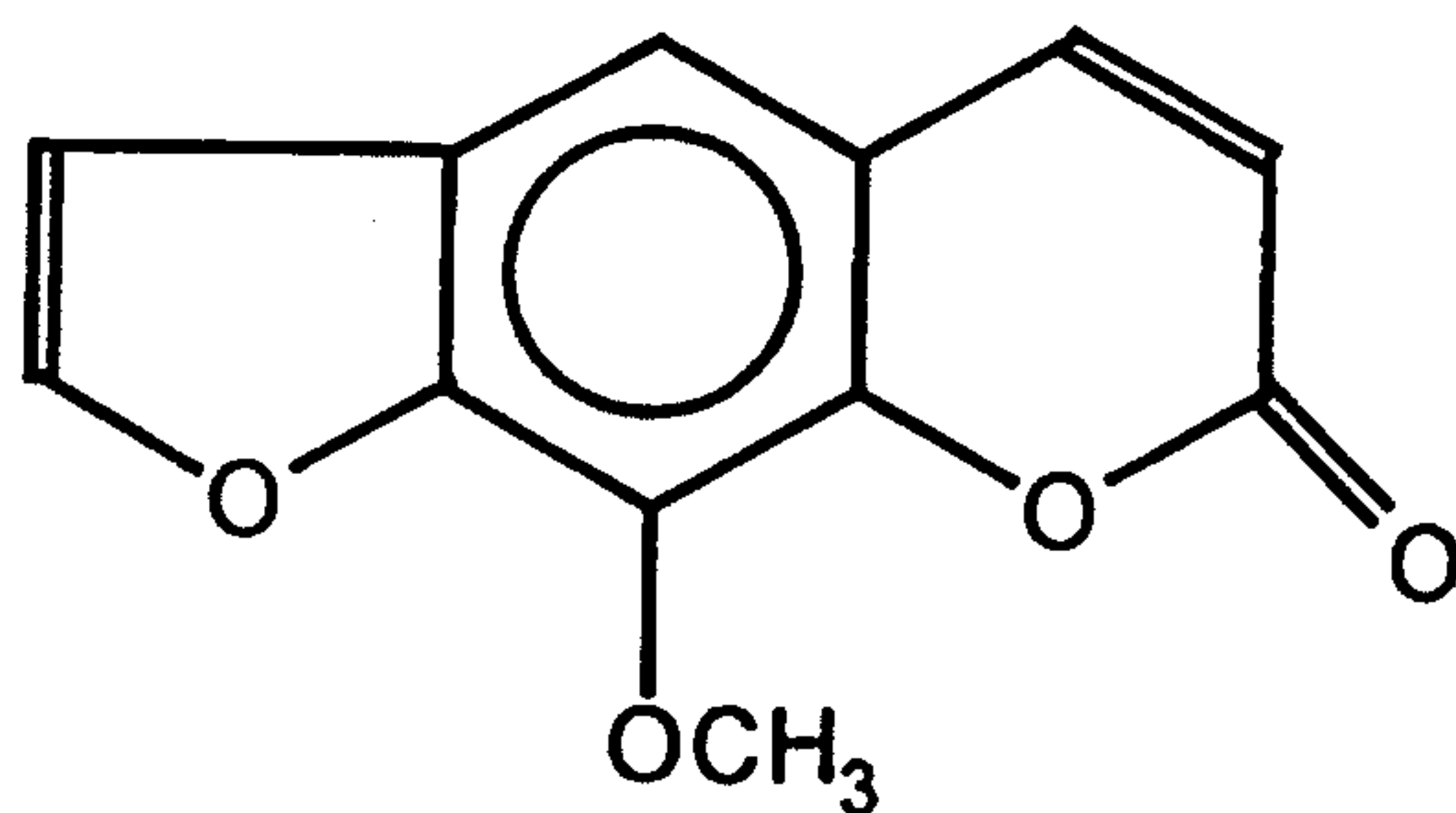
Methoxsalen
