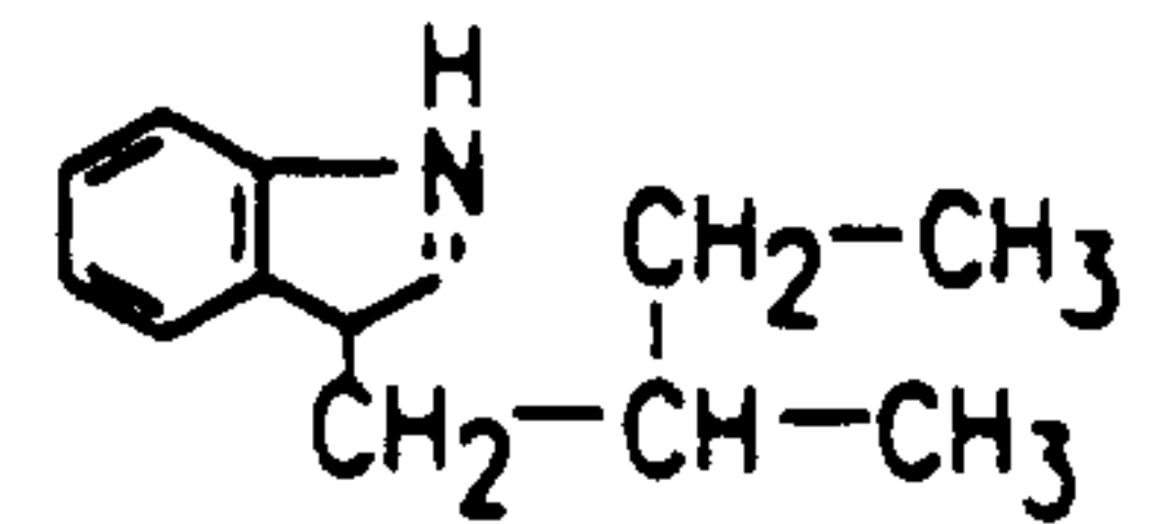
Etryptamine
