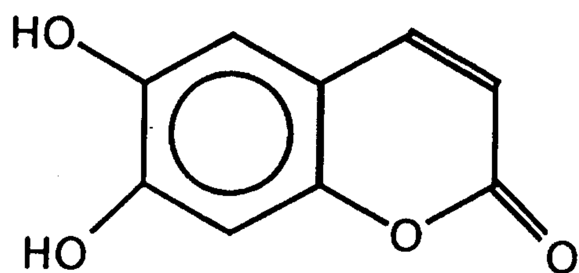
Esculetin
