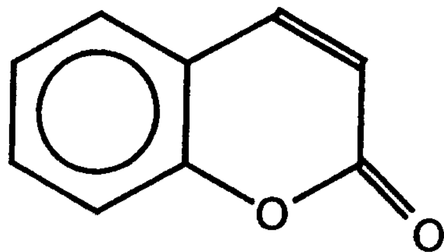
Coumarin
