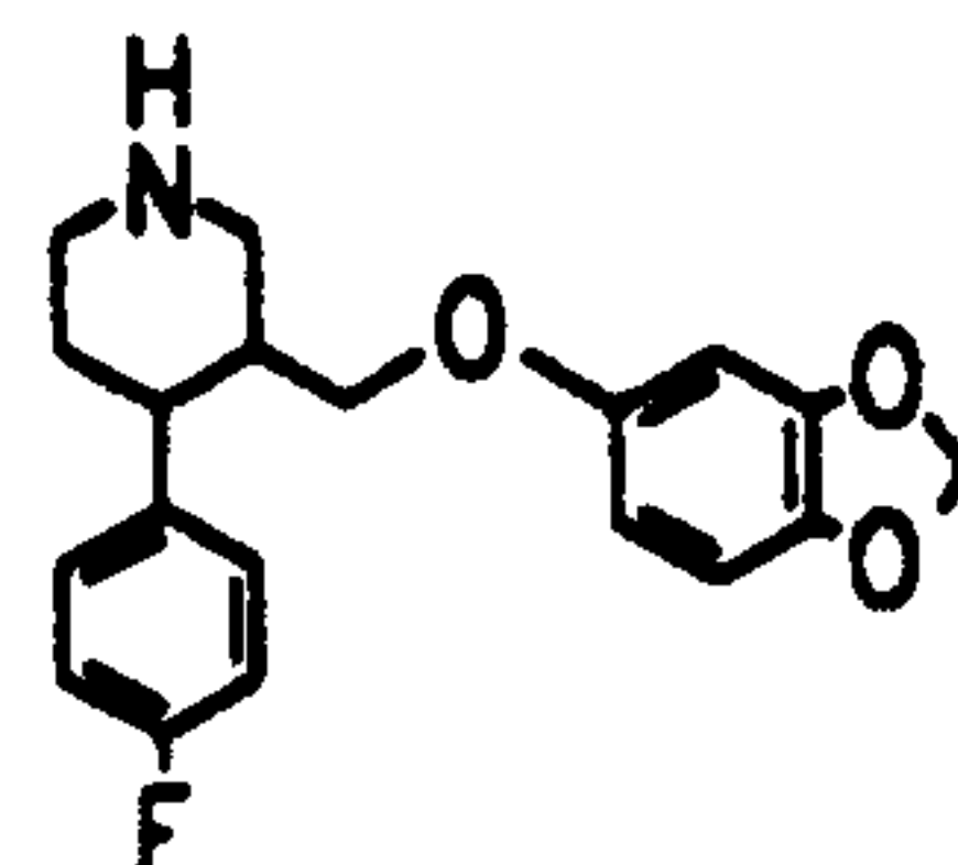
Paroxetine
