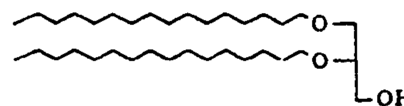
Structure 10. 2,3- Di glycerol
