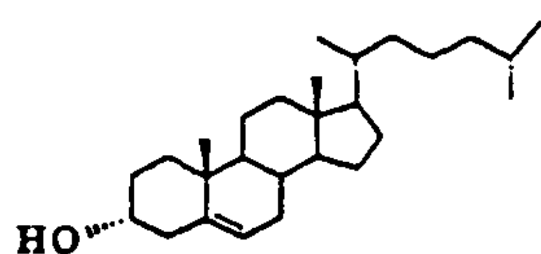
Structure 9. Cholesterol hexadexyl-rac-
