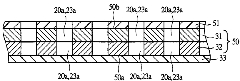
FIG. 9E Resist removing step
