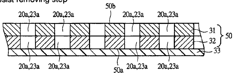
FIG. 9E Resist removing step
