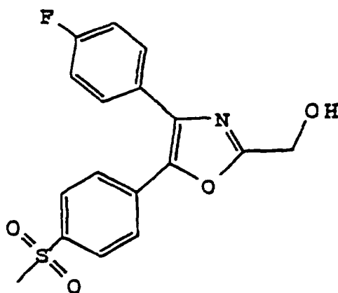
4-(4-Fluorophenyl)-2-(hydroxymethyl)-5-[4-(methylsulfonyl)phenyl]oxazole
