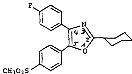
4-(4-Fluorophenyl)-2-cyclohexyl-5-[4-(methylsulfonyl)phenyl]oxazole
