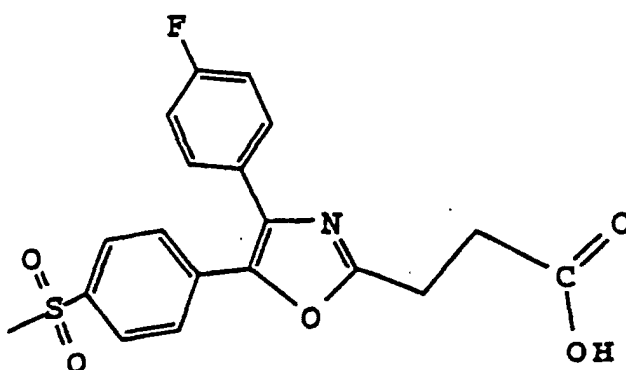
3-[4-(4-Fluorophenyl)-5-[4-(methylsulfonyl)phenyl] oxazol-2-yl]propanoic acid
