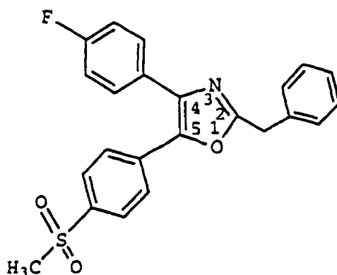
2-Benzyl-4-(4-fluorophenyl)-5-(4-(methylsulfonyl)phenyl)oxazole
