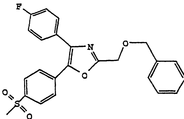
4-(4-Fluorophenyl)-2-benzyloxymethyl-5-[4-(methylsulfonyl)phenyl]oxazole
