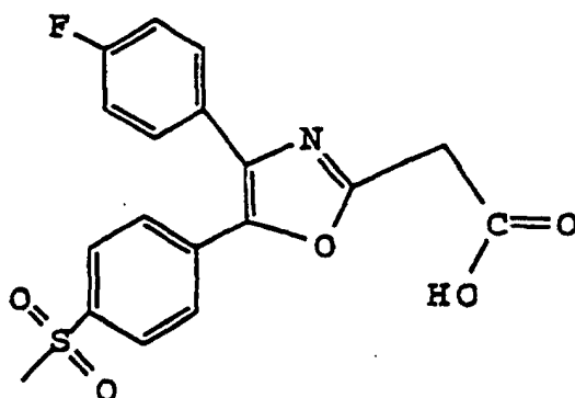
2-[4-(4-Fluorophenyl)-5-[4-(methylsulfonyl)phenyl] oxazol-2-yl]acetic acid
