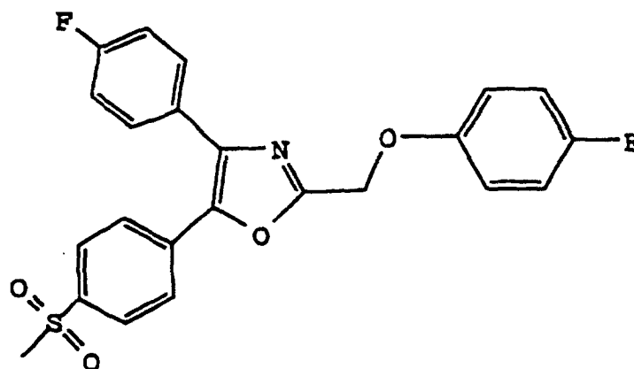
4-(4-Fluorophenyl)-2-(4-fluorophenoxymethyl)-5-[4-(methylsulfonyl)phenyl]oxazole
