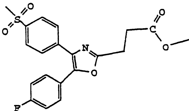
Methyl 3-[5-(4-fluorophenyl)-4-[4-(methylsulfonyl)phenyl]oxazol-2-yl]propanoate
