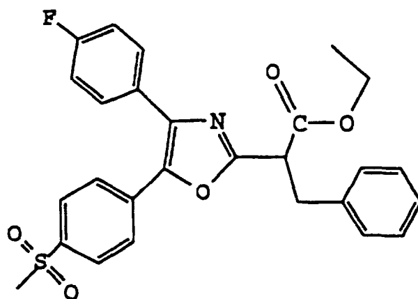
Ethyl 2-[4-(4-fluorophenyl)-5-[4-(methylsulfonyl)phenyl]oxazol-2-yl]-2-benzylacetate
