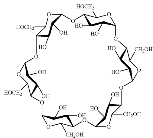
\alpha -Cyclodextrin
