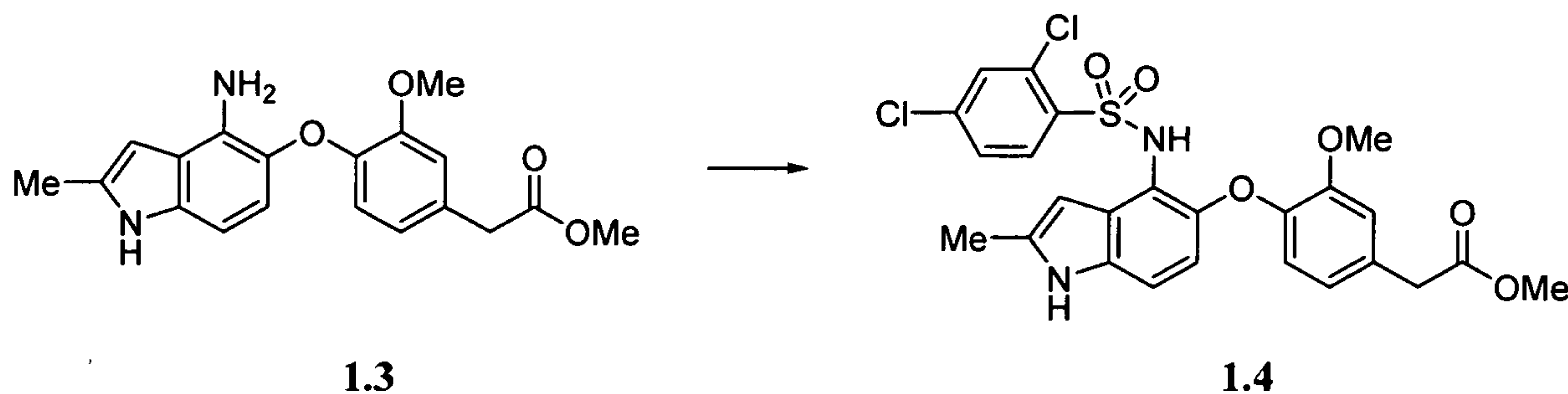
Scheme 1.4
