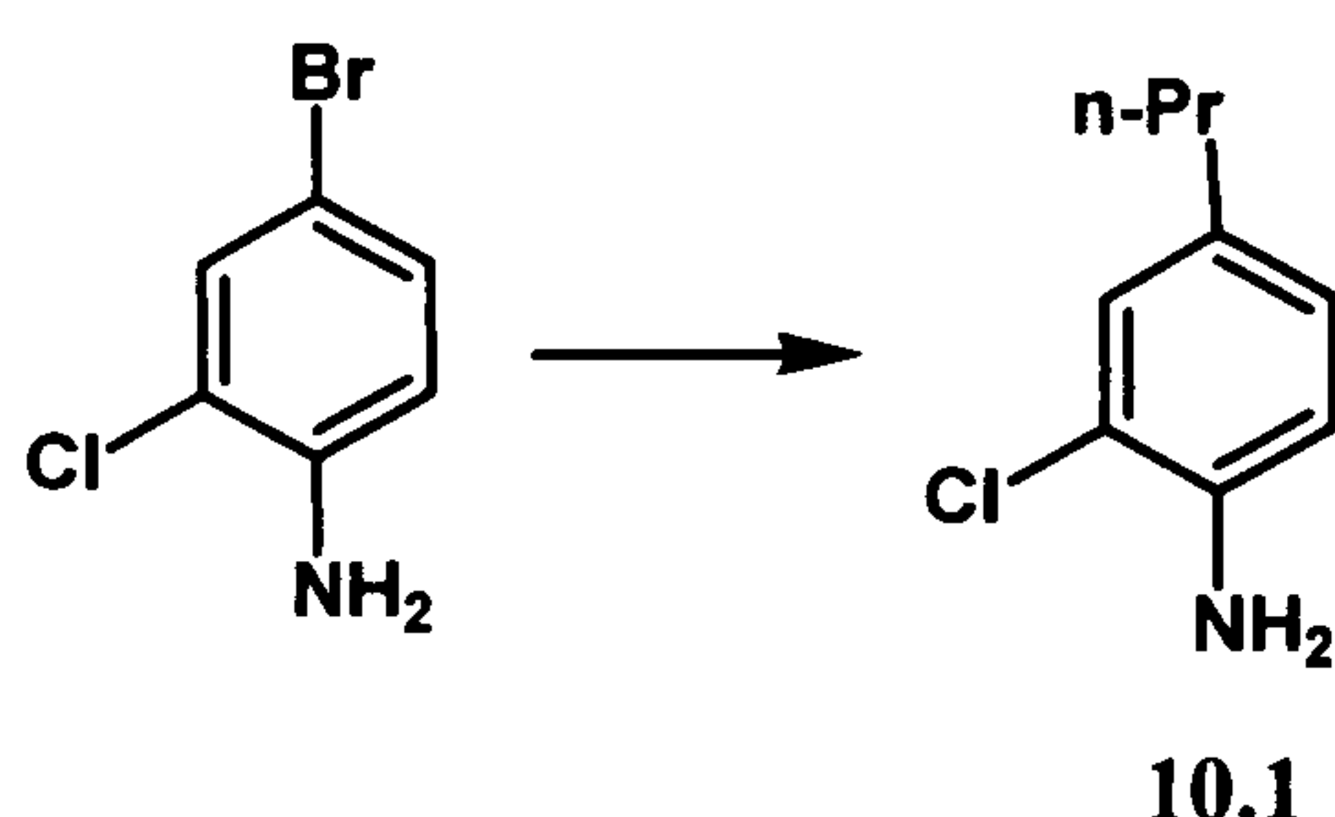
Scheme 10.1
