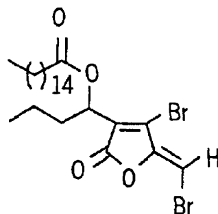
FURANONE 39
