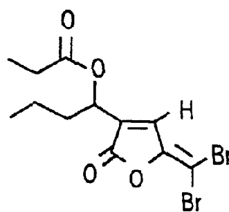
FURANONE 47
