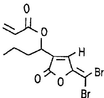
FURANONE 44
