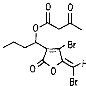
FURANONE 51
