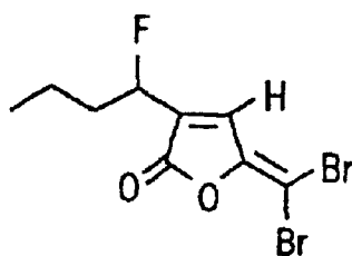
FURANONE 59
