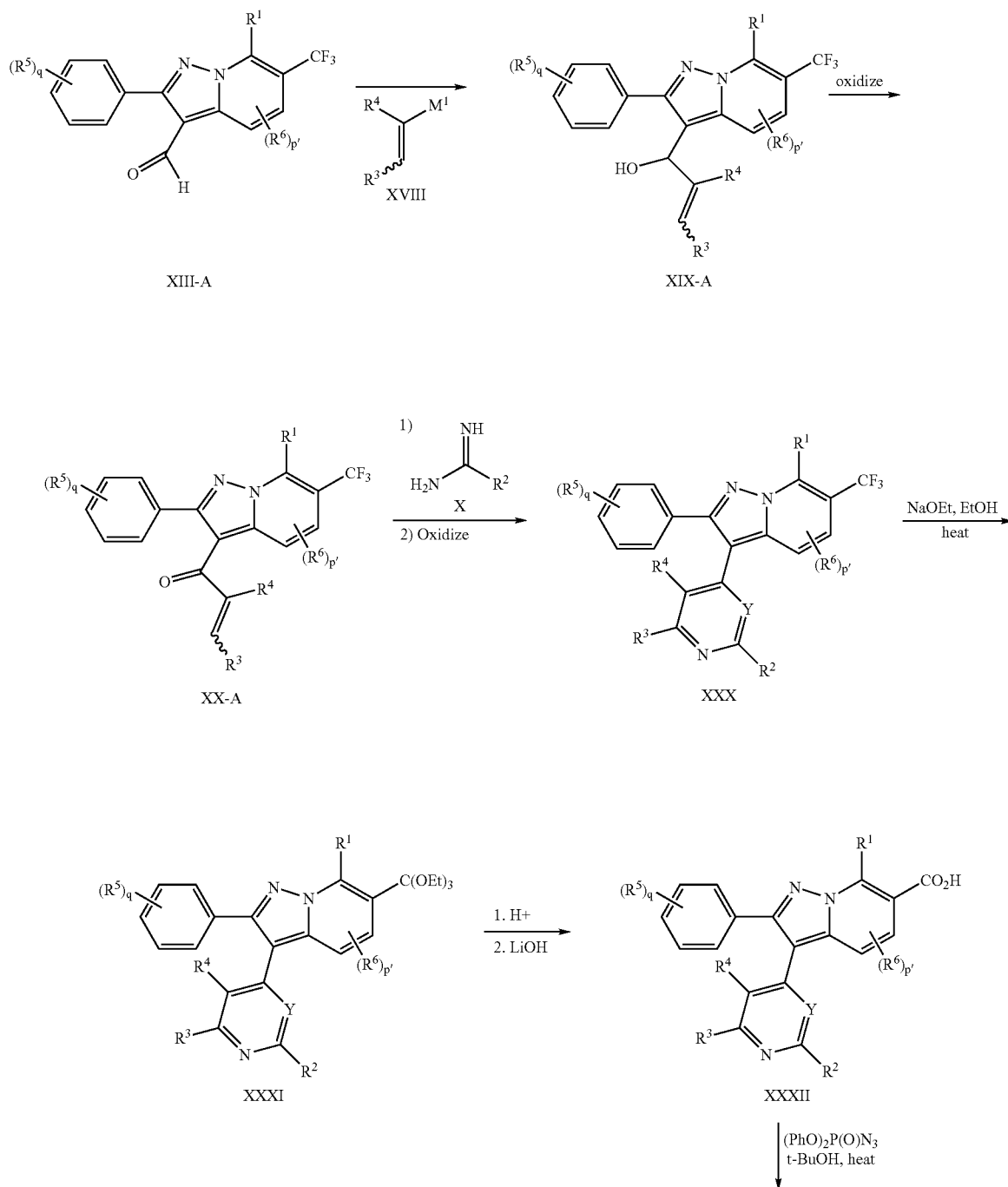
Scheme 3-A
