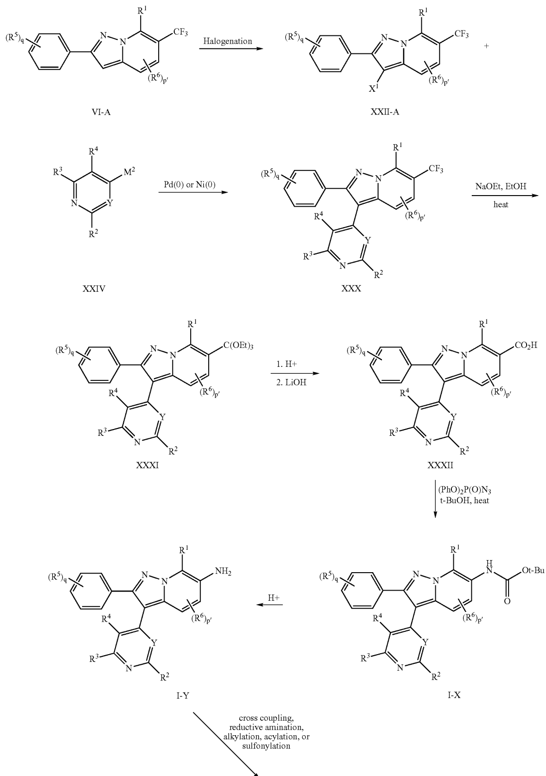
Scheme 4-A
