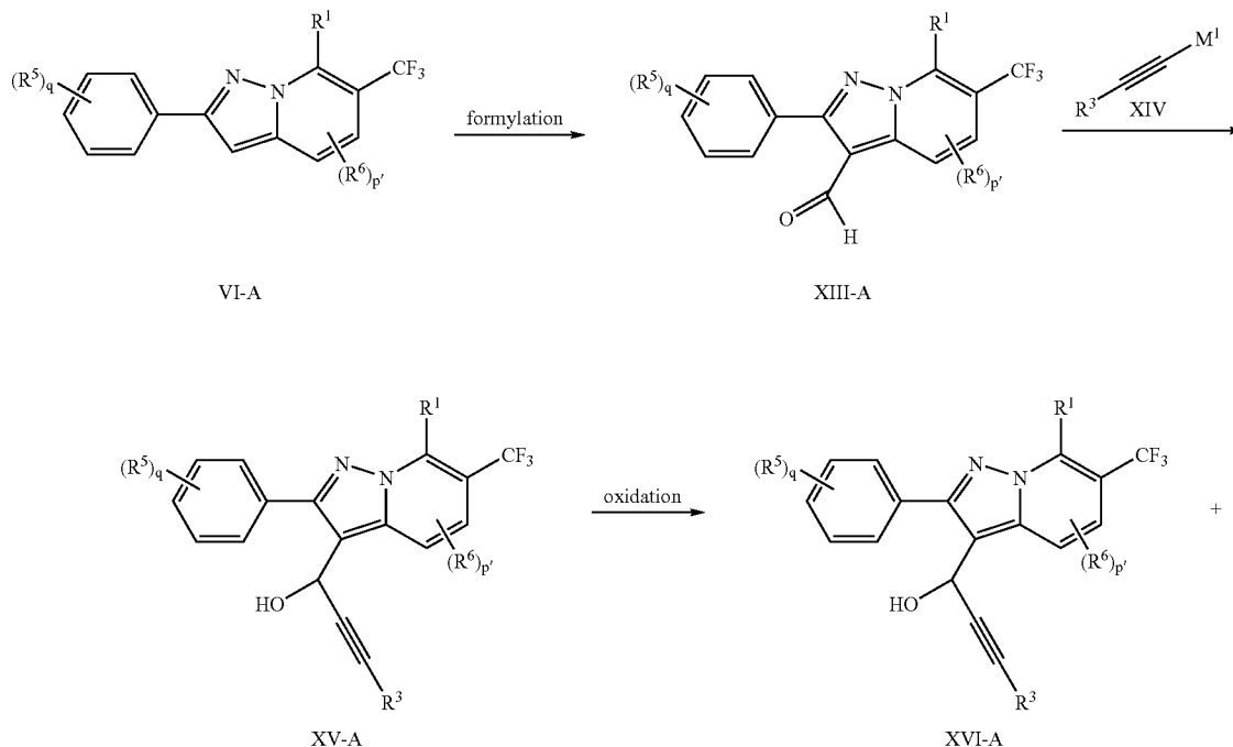
Scheme 2-A
