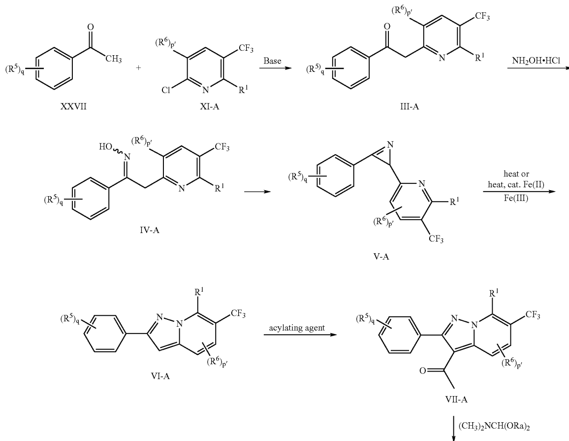
Scheme 1-A
