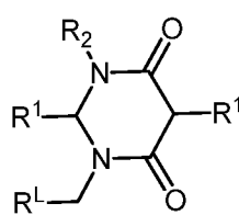
(V-h)
