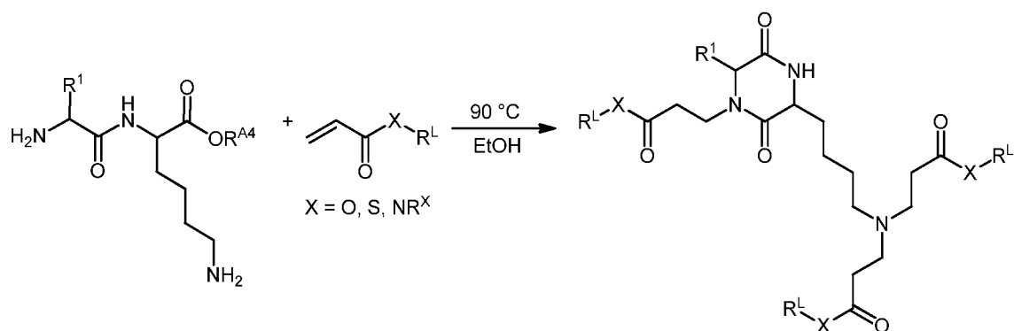
Scheme I.
