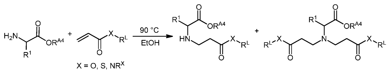
Scheme F.
