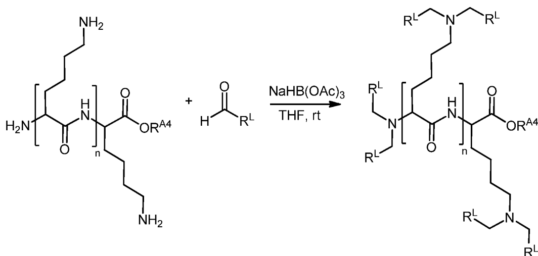
Scheme O.
