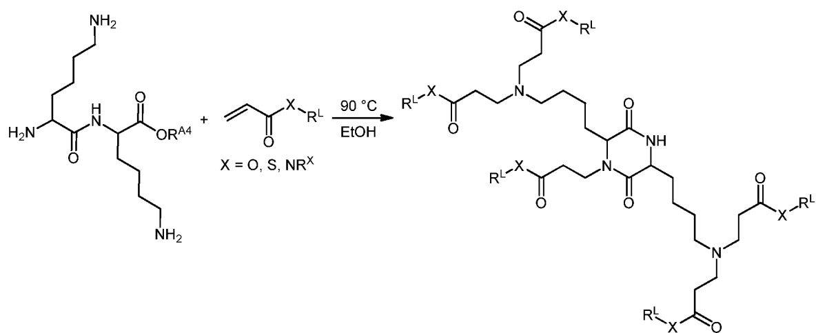
Scheme I.
