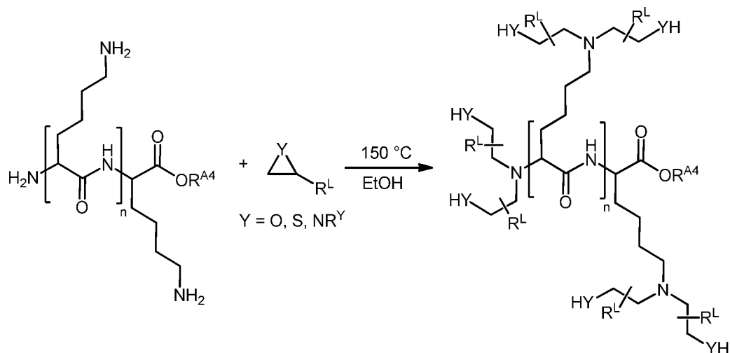
Scheme E.
