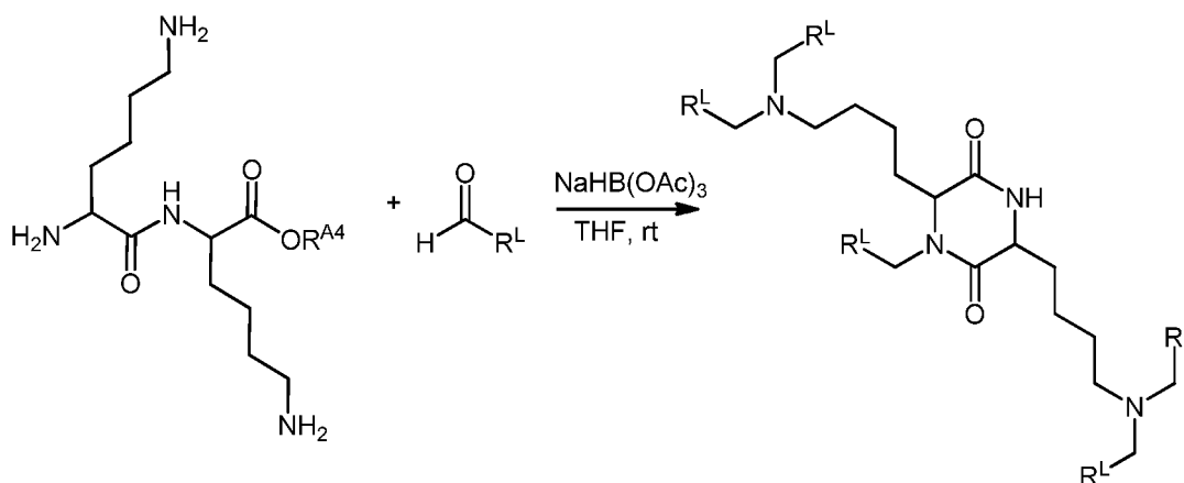
Scheme N.
