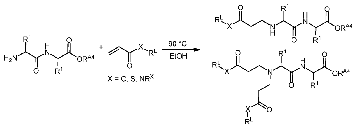
Scheme G.
