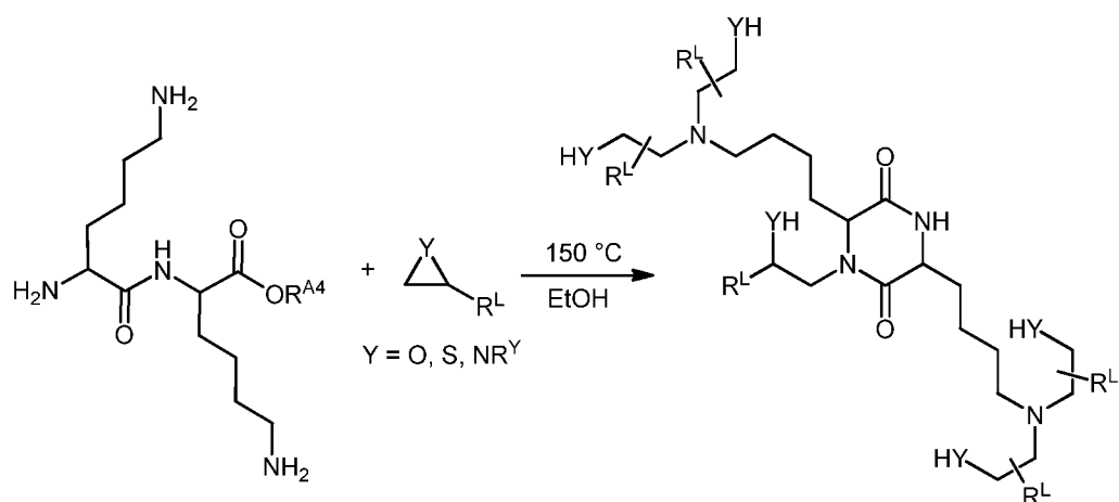
Scheme E.
