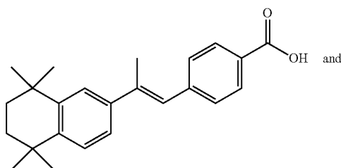
AGN 190183
