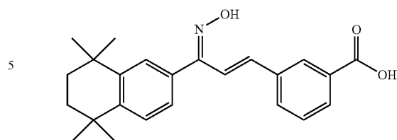
AGN 190183
